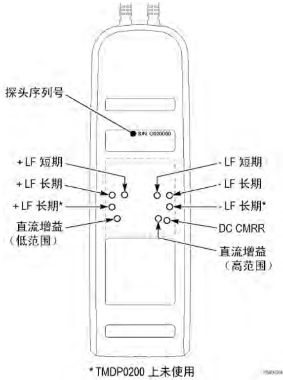
图 13: 探头序列号及调节位置
