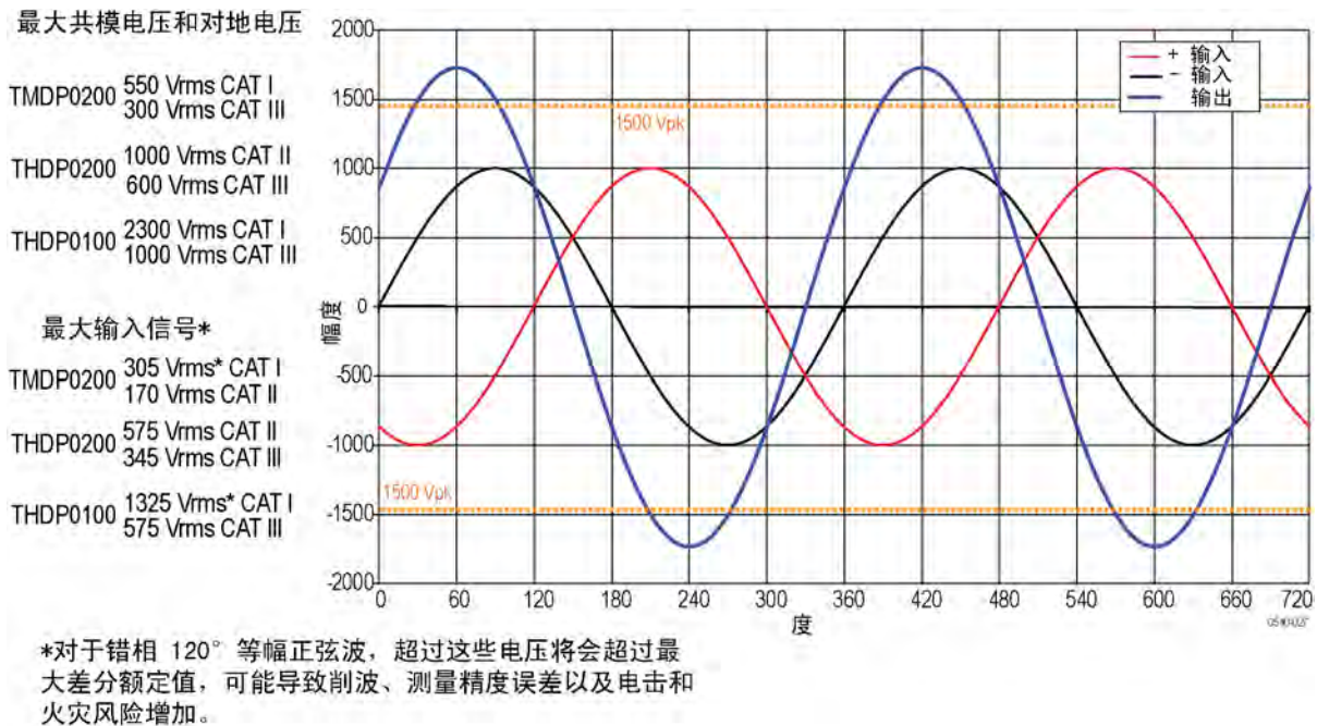
图 4: 测量两个错相 120 度的等幅波形
