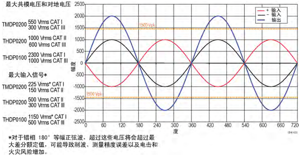
图 3: 测量两个错相 180^\circ 的等幅波形
