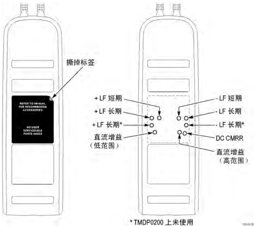
图 14: 内部调节位置 (仅序列号 C020000 及以上)
