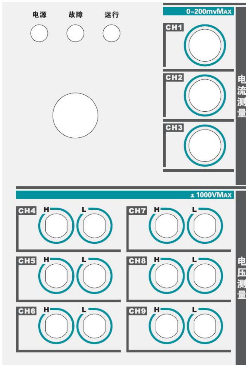
前面板电压、电流采集测量接线示意图
