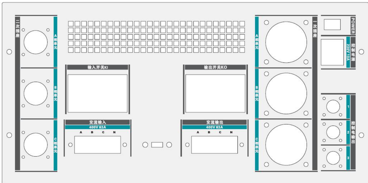
电压扰动发生装置控制模块前视图
