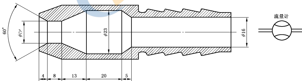
图 D.4 标准的喷水法(软管法)试验滴嘴
