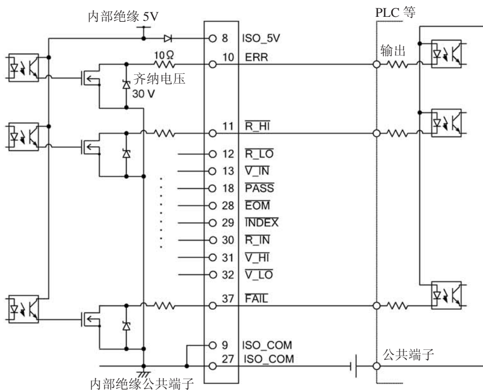
输出电路
