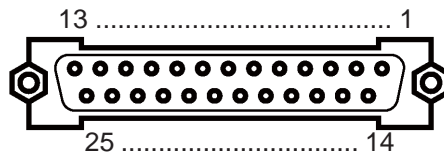
打印机（25 针）连接器（例）
