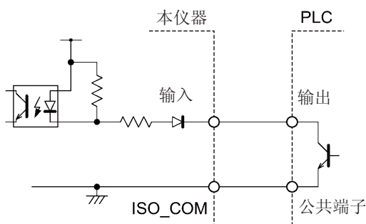
与 PLC 输出（负公共端子输出）的连接
