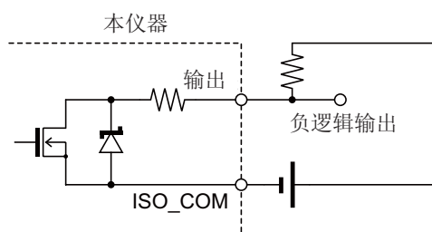
负逻辑输出
