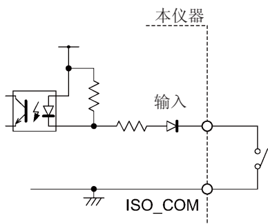
与开关的连接
