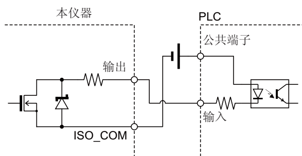
与 PLC 输入（负公共端子输出）的连接
