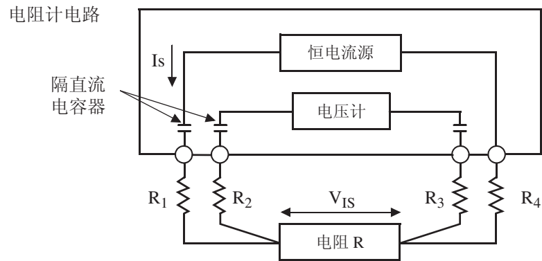
R_1 \sim R_2 : 测试线的电阻和接触部分的接触电阻
