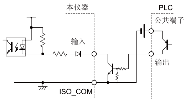
与 PLC 输出（正公共端子输出）的连接
