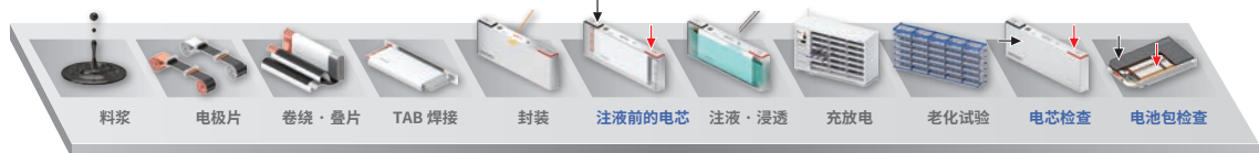
锂电池生产线的工序示意图
