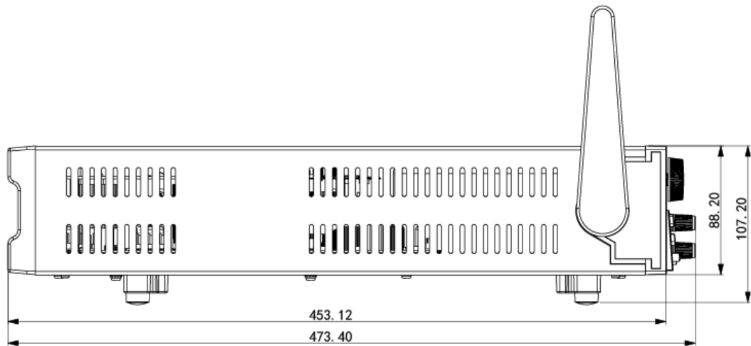
IT6332L 侧面图
