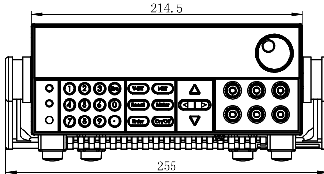
IT6332L 前视图
