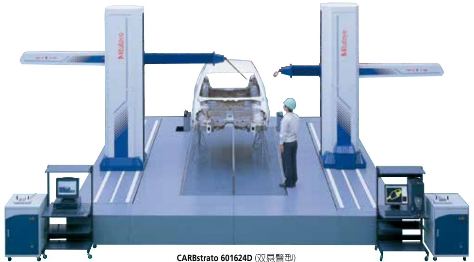
CARBstrato 601624D (双悬臂型)
