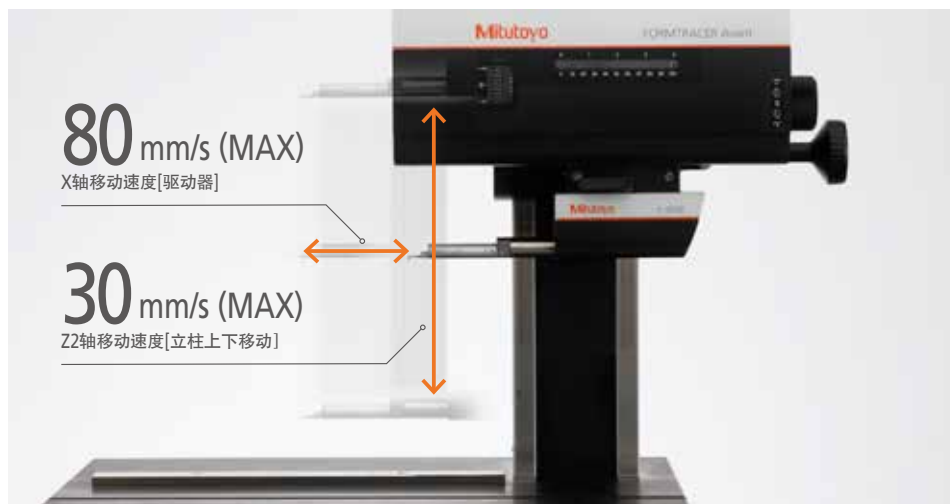
X轴(驱动器): 80mm/s(MAX) Z轴(立柱上下移动): 30mm/s(MAX) 通过提高移动速度缩短总测量时间。
