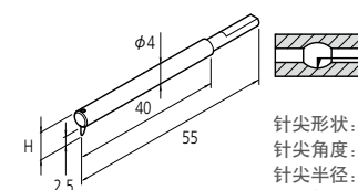
小孔测针 SPH-43
