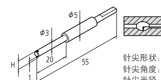
小孔测针 SPH-42
