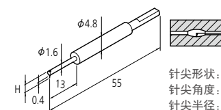
小孔测针 SPH-41
