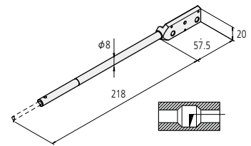
小孔测臂 AB-33
