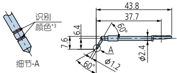
滚动圆波表面测针*4
