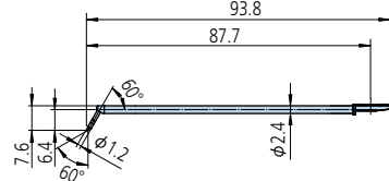
孔测量拐角用/深孔2倍长测针 *2
