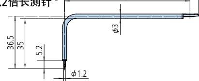
齿面测针 深孔2倍长测针 *2
