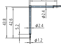
深槽测针(30mm) 深孔2倍长测针 *2
