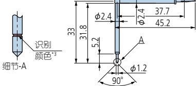
齿轮齿面测针
