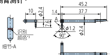
偏心测臂测针 *2
