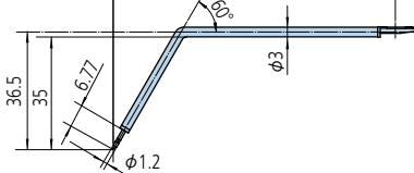
滚动圆波表面测针/深孔2倍长测针 *2 *4
