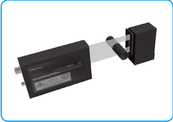
胶辊外径测量
