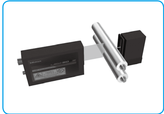
辊子缝隙的测量
