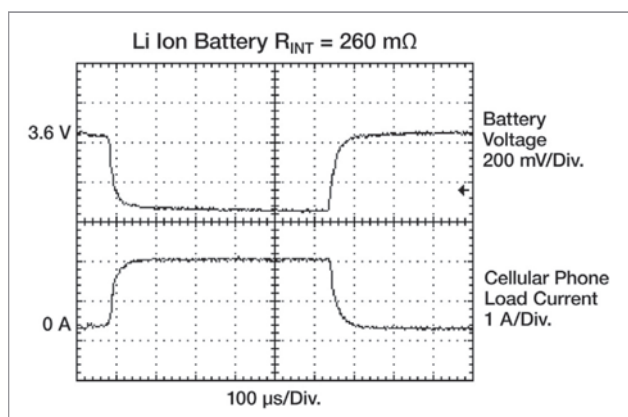
图 2. 锂离子电池 (内阻 260mΩ) 与 2306 型电池通道 (输出电阻可设置为 260mΩ) 输出电压比较。当为蜂窝电话供电时, 电池从待机模式转为传输模式。
