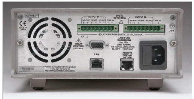
图 9. 2306-LAN 后面板
