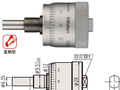
质量: 103g 148-311-10 MHC1-13GA 微分筒直径 \phi 29
