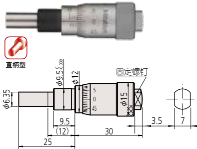
质量: 35g 148-307-10 MHC1-13CA 微分筒直径 \phi 15
