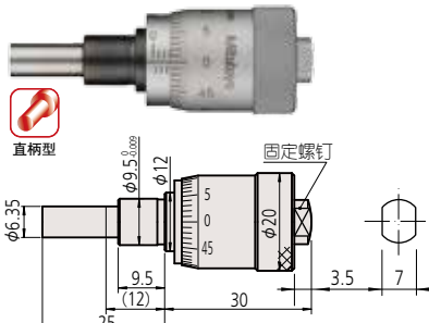
质量: 55g 148-309-10 MHC1-13MA 微分筒直径 \phi 20
