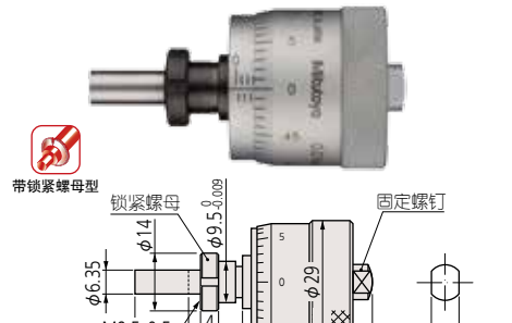
●固定装置厚度: 6mm 质量: 103g 148-312-10 MHC2-13GA 微分筒直径 \phi 29
