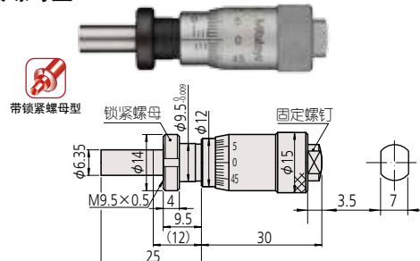
●固定装置厚度: 6mm 质量: 35g 148-308-10 MHC2-13CA 微分筒直径 \phi 15
