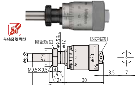
●固定装置厚度: 6mm 质量: 55g 148-310-10 MHC2-13MA 微分筒直径 \phi 20
