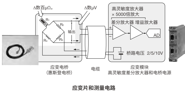
应变片和测量电路
