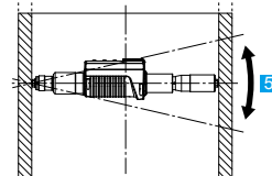
图2 侧视图
