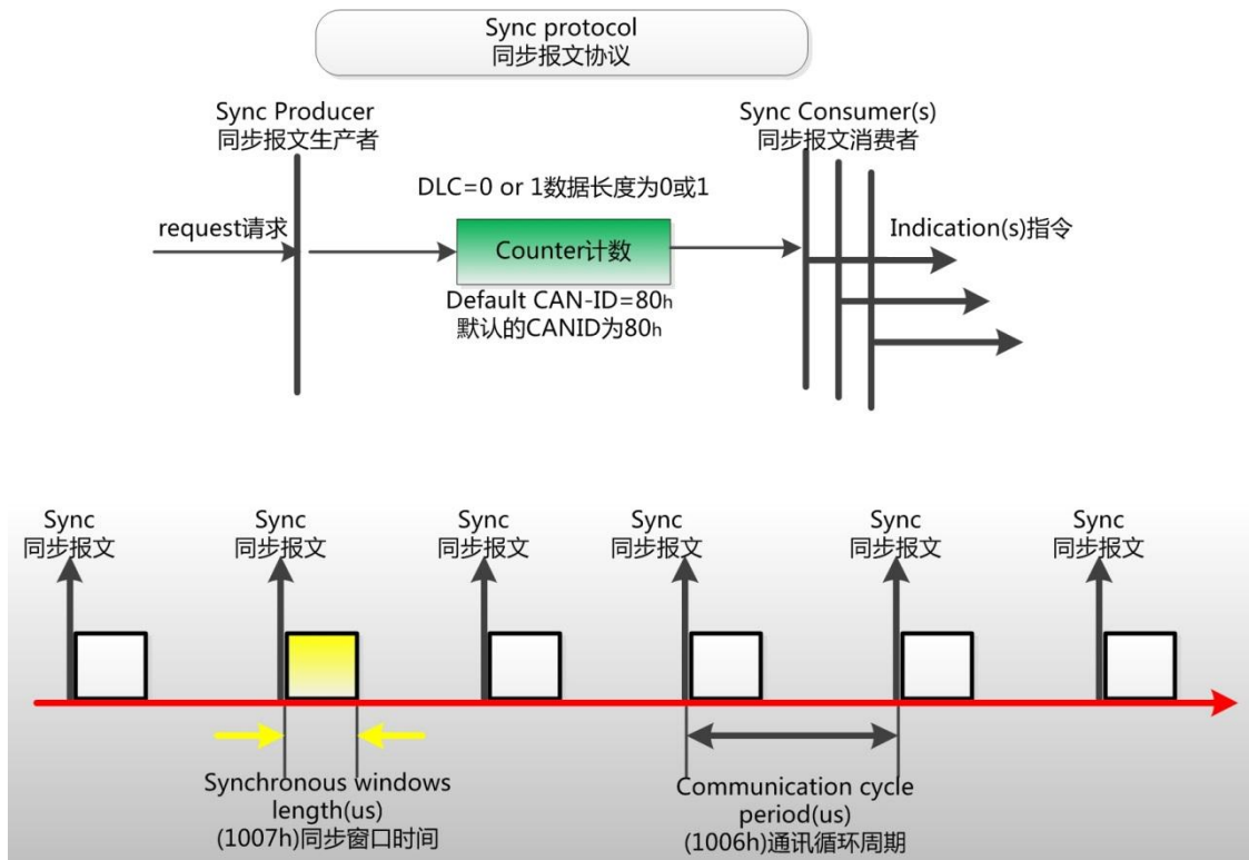
图 9.2 同步报文
