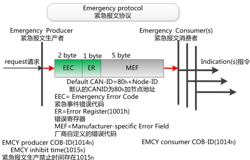
图 9.5 紧急报文
