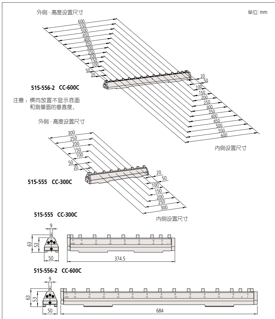
内量爪精度检查
