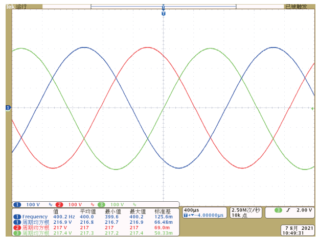
三相相位差120°
