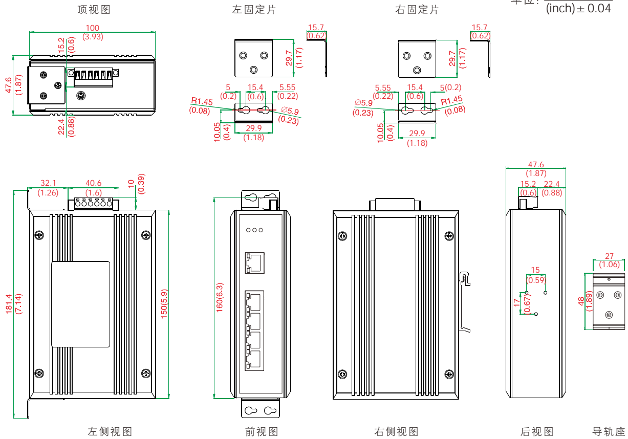
壁挂式安装
