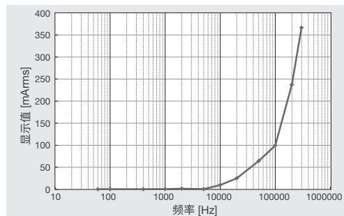
CMRR特性 (例) *
