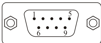
DB9针型
