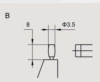
测量壁厚
