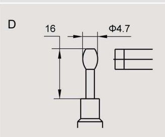
测量深孔壁厚
