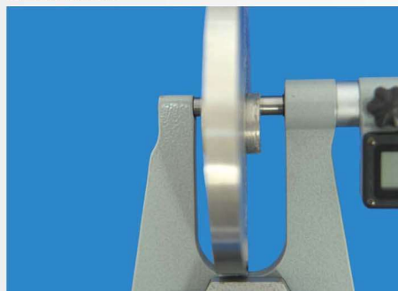
测量轮毂厚度
