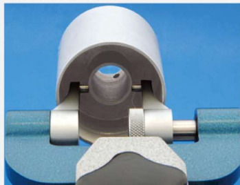
测量内台阶尺寸
