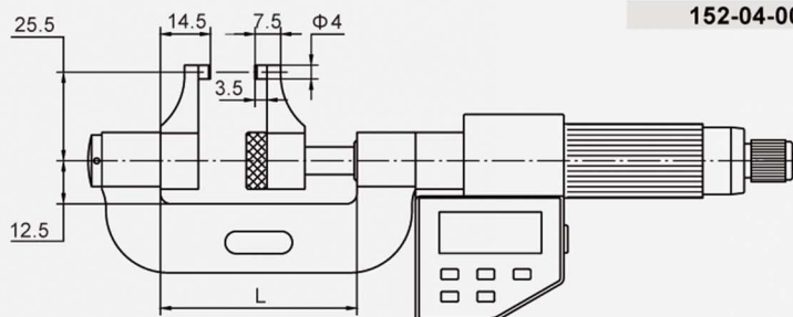
测量内台阶尺寸
