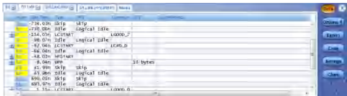
总线协议的表格视图。结果表格提供了总线的协议视图, 通过鼠标单击可将物理层的事件与协议层的事件关联起来。
