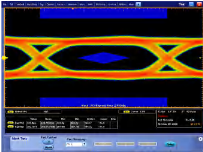
通信模板测试。
