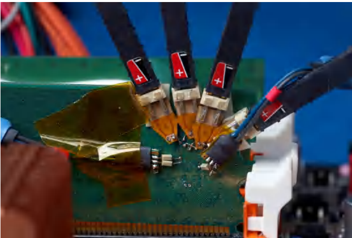
为 P6780 差分逻辑探头设计的焊接式探头尖端附件，提供了在小间距过孔和紧密排列的器件上访问信号的能力。
