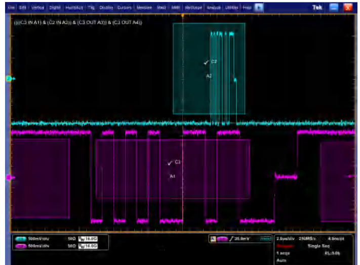
多条通道触发。可视触发区域可以与跨越多条通道的事件相关，如两条 USB 2.0 总线上同时传送的数据包。
