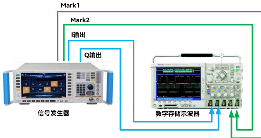
图 4.23 触发测试
