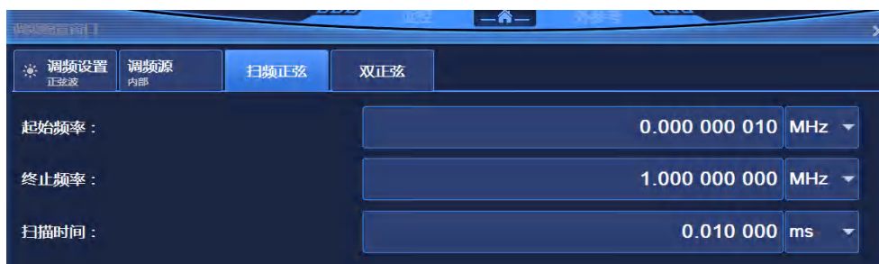
图 5.21 扫频正弦界面
