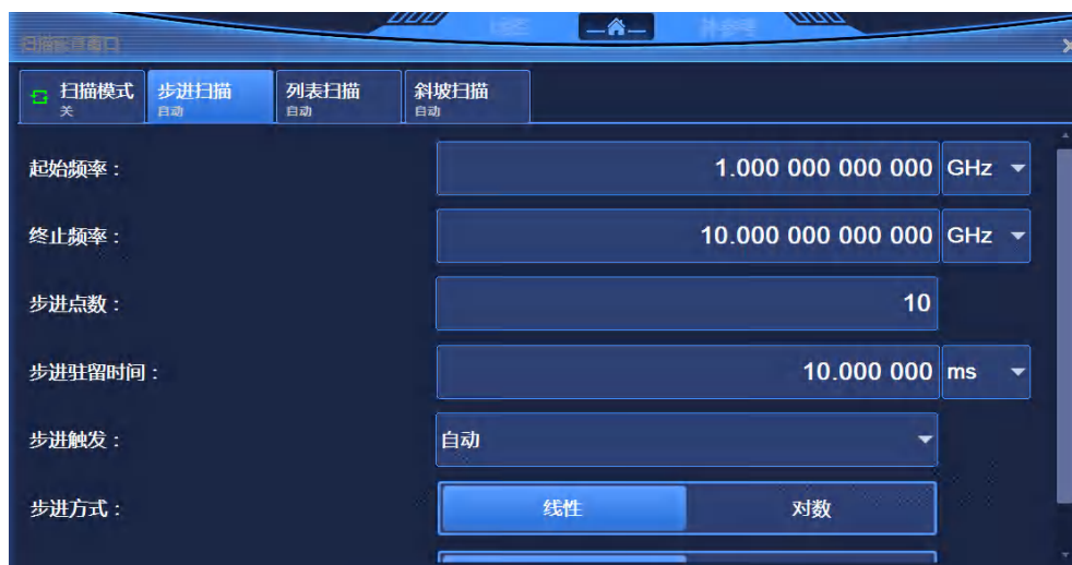
图 4.5 步进扫描配置窗口
