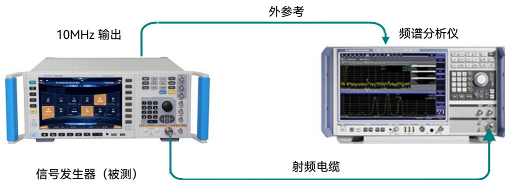
图 8.6 小功率测试
