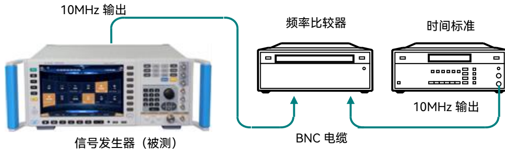
图 8.3 内部时基老化率测试
