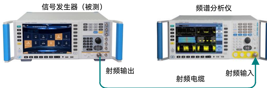
图 8.4 谐波测试
