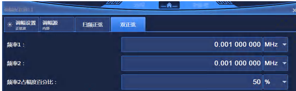
图 5.18 双正弦界面
