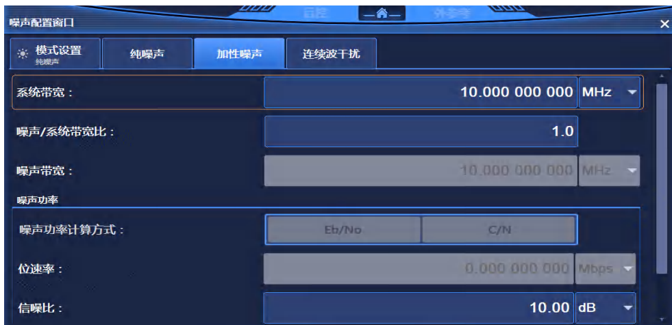
图 5.48 加性噪声界面
