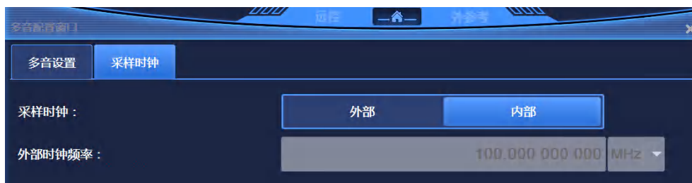
图 5.45 采样时钟界面
