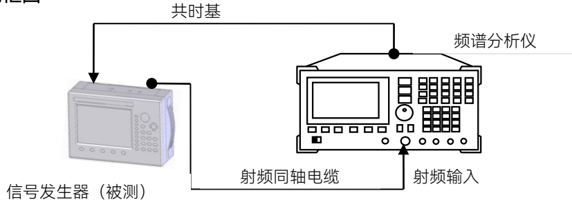
图 7-3 谐波寄生测试
