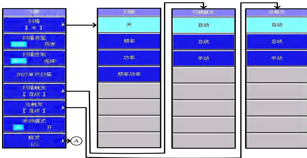
图 5-5 扫描菜单结构-1
