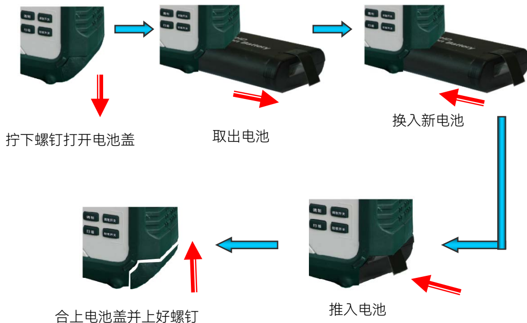
图 3.6 1431A 手持式射频信号发生器电池更换图解
