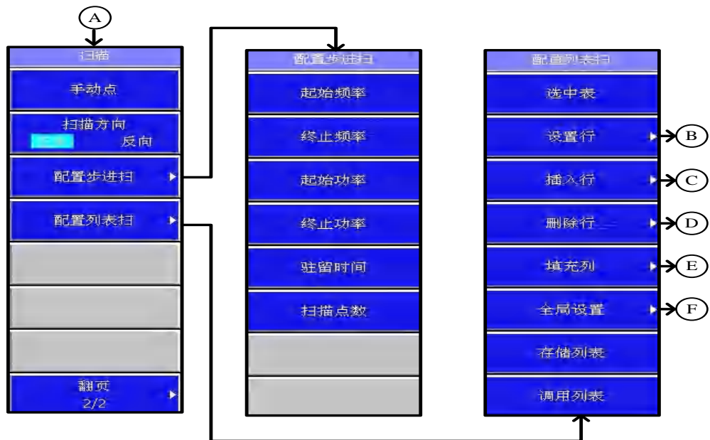
图 5-5 扫描菜单结构-1
