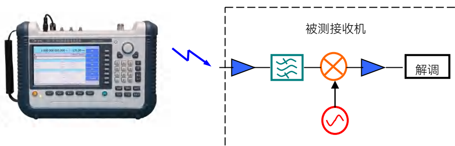
图 2.3 1431A 在高性能接收机测试中的应用
