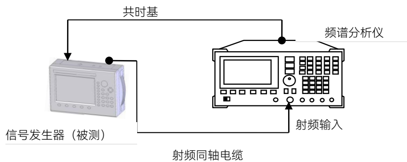
图 7.7 脉冲调制开关比测试框图
