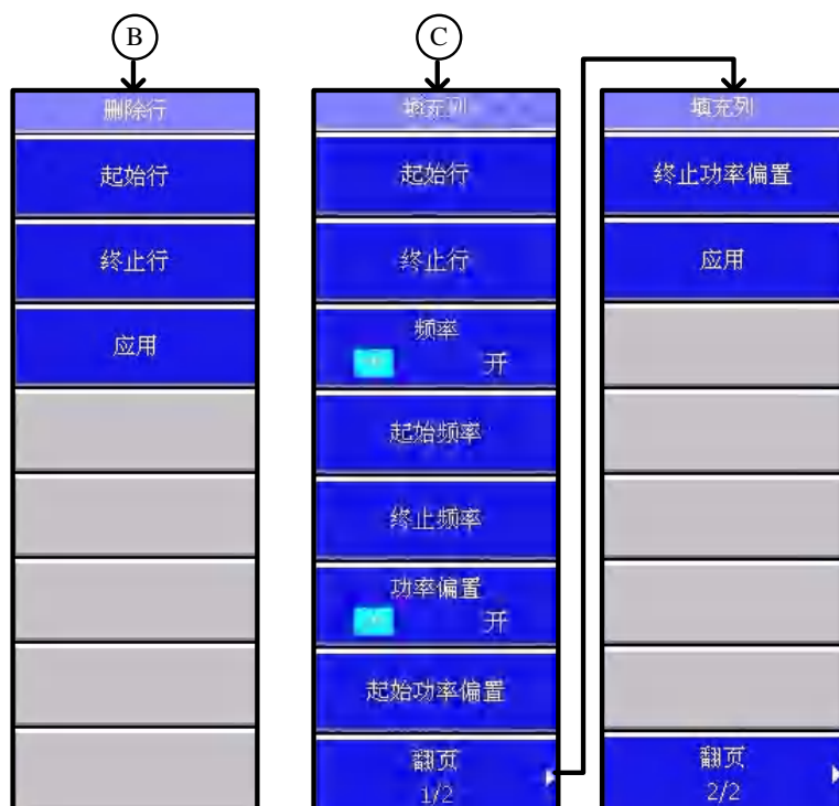
图 5-4 功率菜单结构-3
