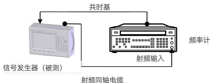
图 7.2 频率分辨率测试框图
