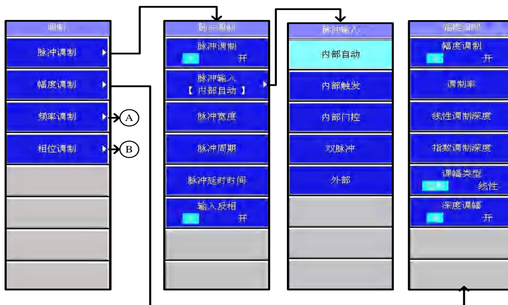
图 5-9 调制菜单结构-1
