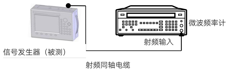
图 7.1 频率范围测试框图
