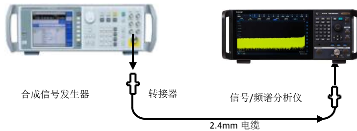
图 7.3 剩余调频测试示意图
