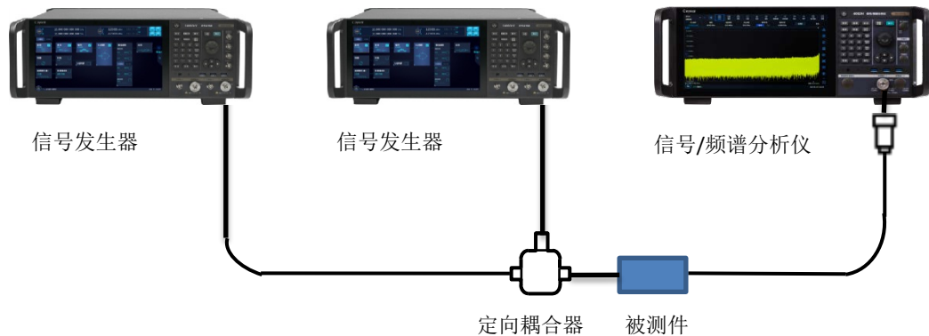
图 4.24 三阶交调测量连接设置
