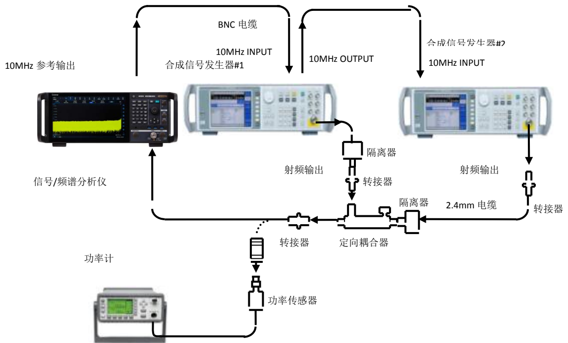
图7.16 三阶交调失真测试示意图 (4GHz ~ 67GHz)
