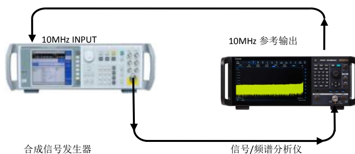
图 7.4 标记计数测试示意图
