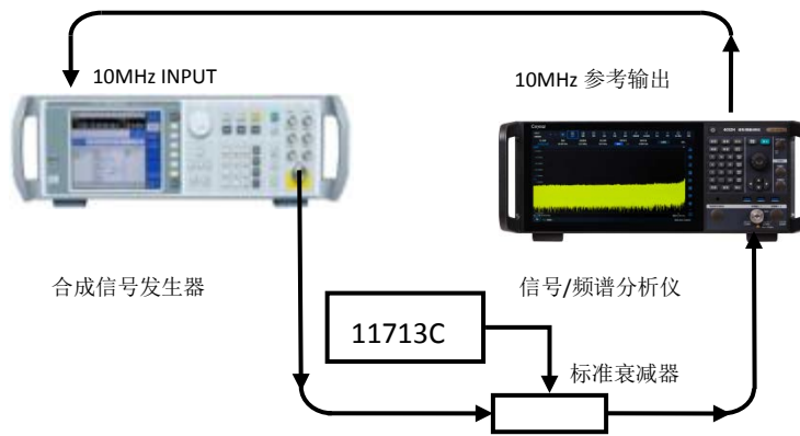
图7.11 参考电平转换误差测试示意图
