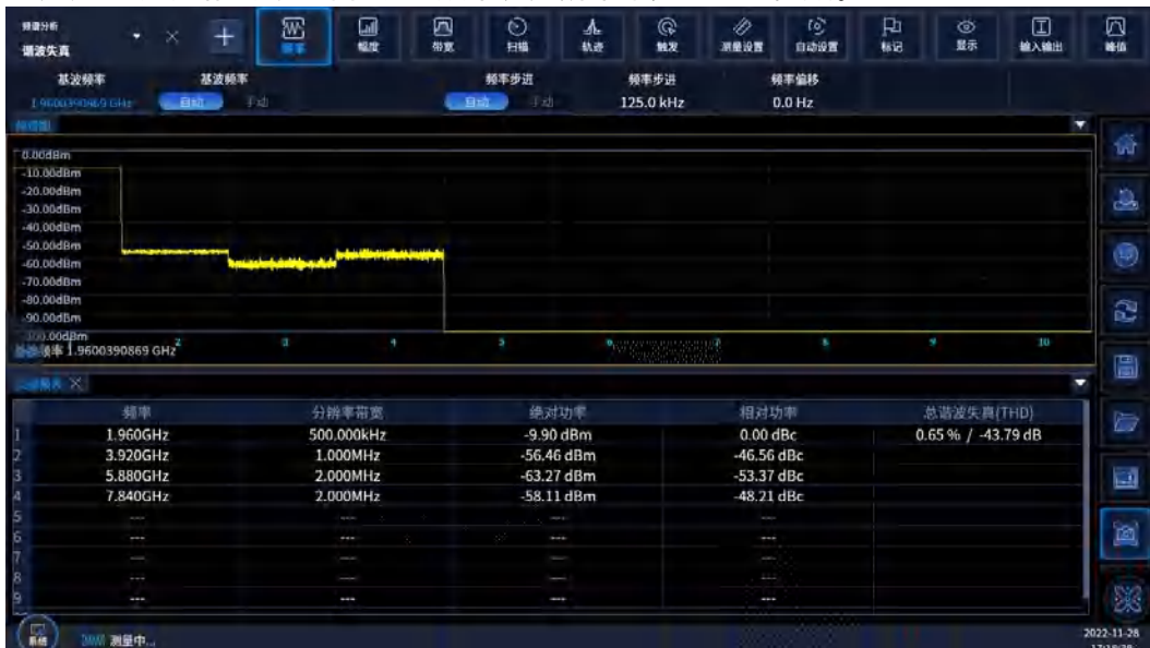
图 4.23 谐波失真测量结果
