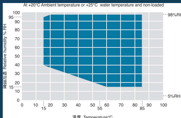
溫濕度控制範圍梯形圖
