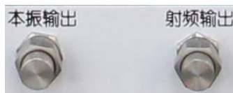
图3.27 本振和射频输出连接器
