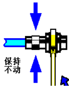
图 3.6 使用力矩扳手完成最后连接
