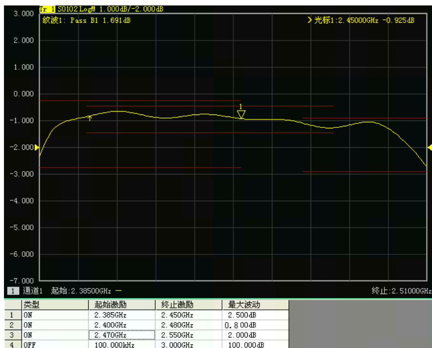
图 3.53 纹波测试结果
