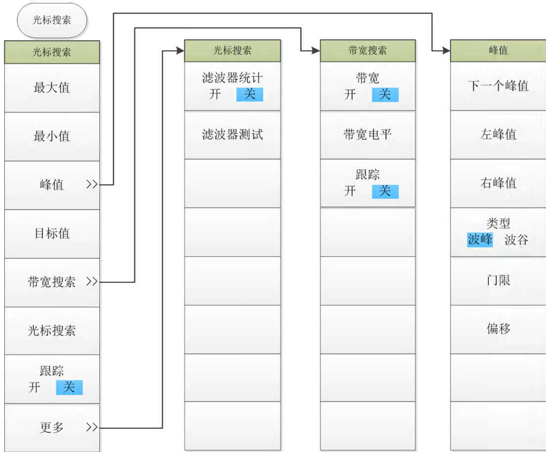
图 5.14 光标菜单二
