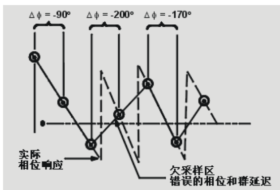
图 7.15 欠采样对群时延测量的影响
