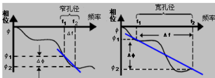
图 7.14 群时延孔径对测量结果的影响
