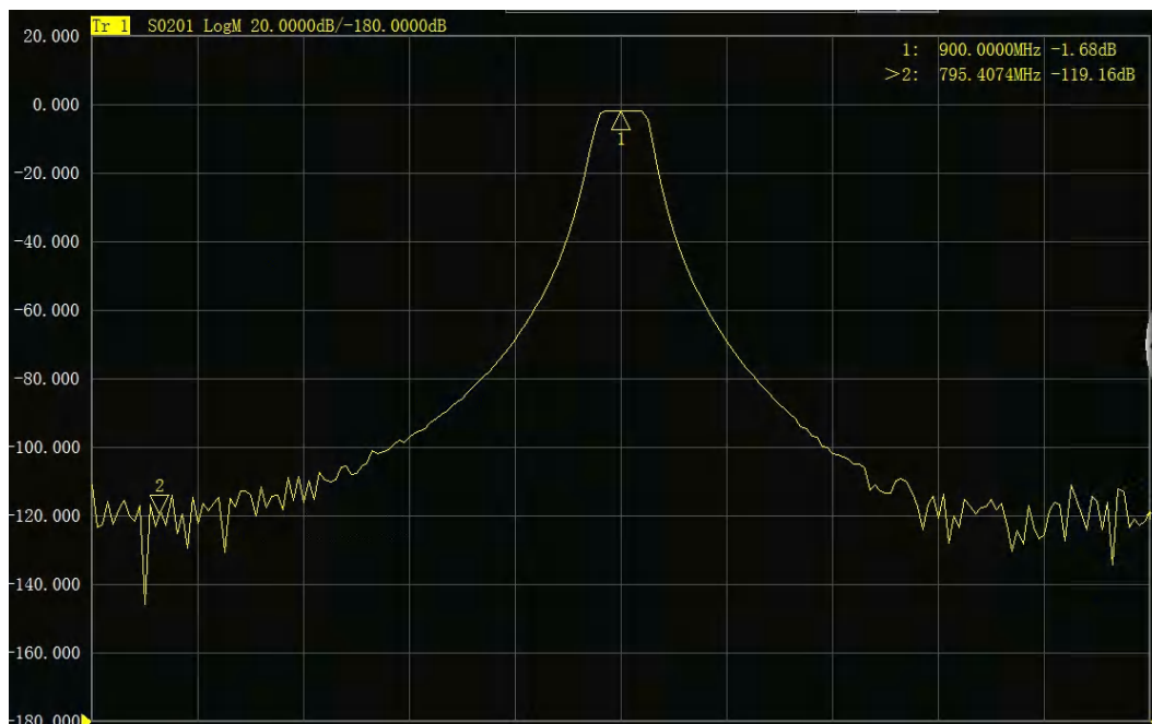
图 2.5 滤波器测量结果
