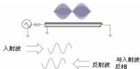
图7.3 用短路器端接的传输线的信号传输
