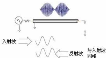
图 7.4 用开路器端接的传输线的信号传输
