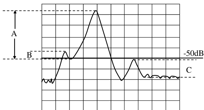
图 3.40 光标域内峰值示意图
