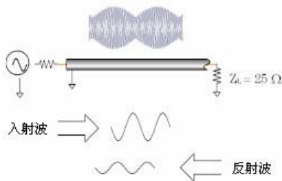
图 7.5 用 25\Omega 电阻端接的传输线的信号传输
