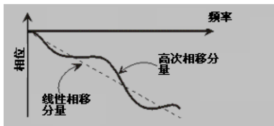
图 7.11 相移与群时延
