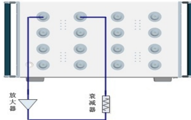
图 7.16 群时延测量连接
