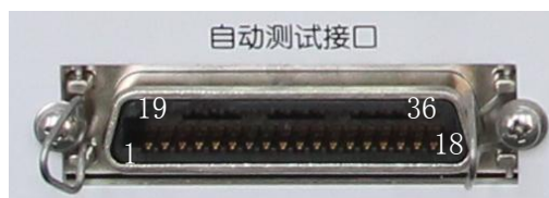
图3.29 自动测试接口连接器
