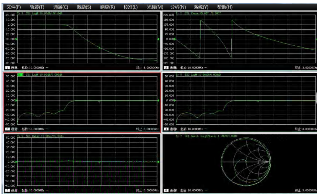
图 2.4 多窗口多通道测量显示
