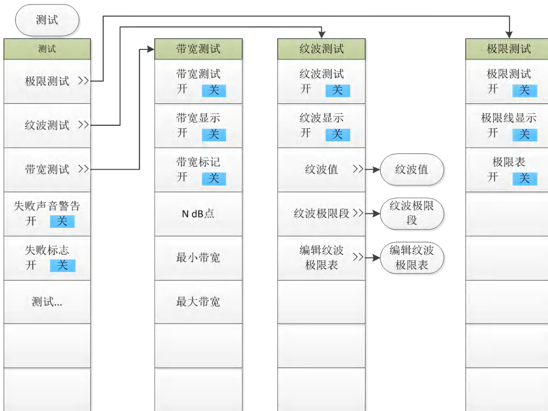
图 5.17 分析菜单二
