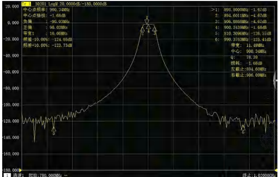
图 3.41 带宽搜索
