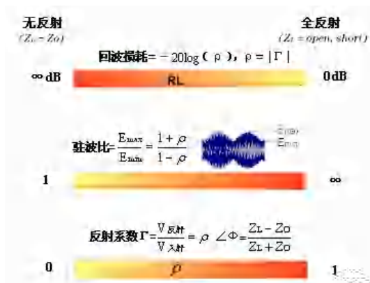
图7.6 各种反射表达之间的关系
