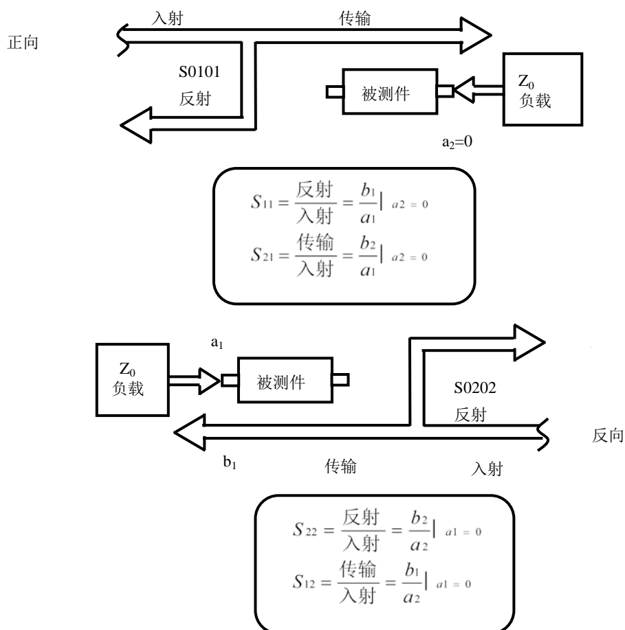
图 4.2 S 参数定义
