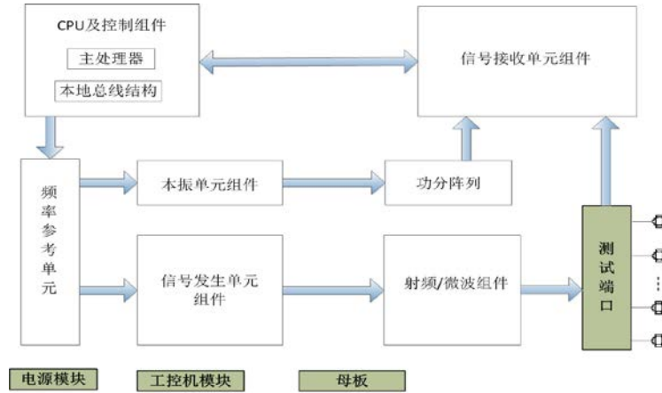
图 8.2 整机原理框图
