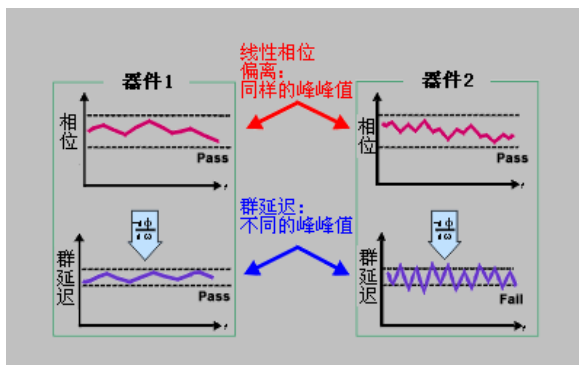
图7.13 群时延与线性相位偏离比较
