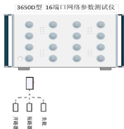
图 9.7 单端口校准连接框图
