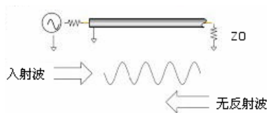
图 7.2 用负载端接的传输线的信号传输
