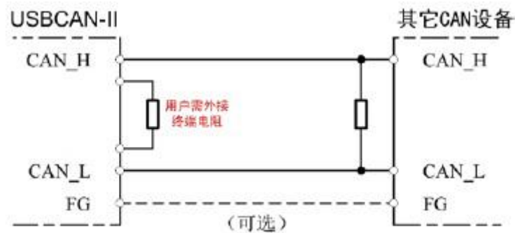
图 3.2 USBCAN-II Pro 与其他 CAN 节点设备连接
