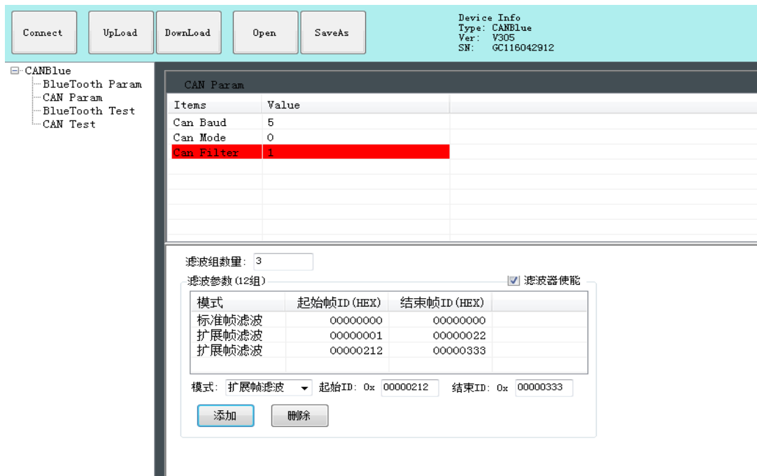
图 4.5 CAN 滤波模式设置
