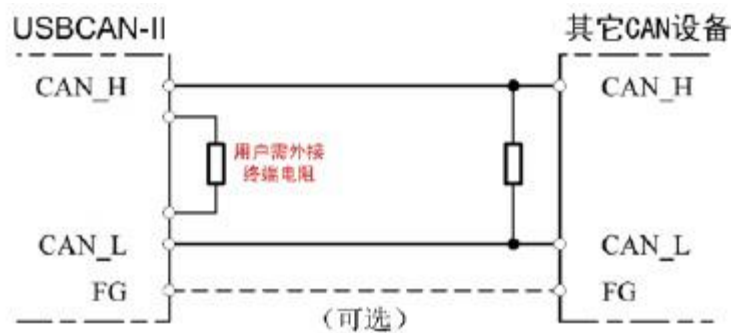
图 3.2 GCAN-203 与其他 CAN 节点设备连接
