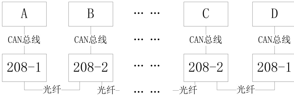
GCFAN-208-2 典型应用——手拉手级联
