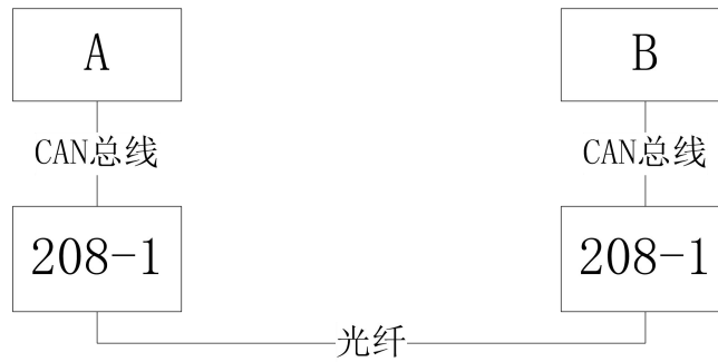
GCFAN-208-1 典型应用——成对使用
