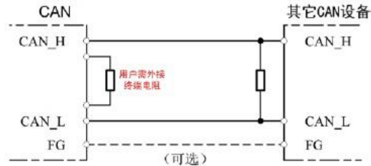
图 3.8 GCFAN-208 系列模块与其他 CAN 节点设备连接
