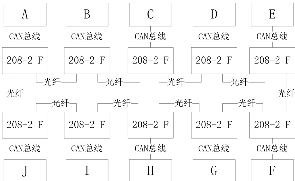
GCFAN-208-2 F 典型应用——环网
