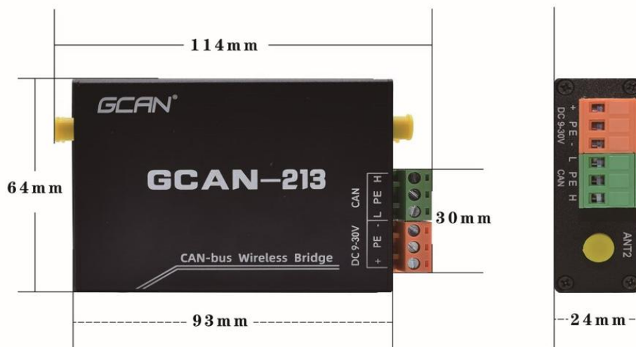
图 2.1 GCAN-213 外形尺寸
