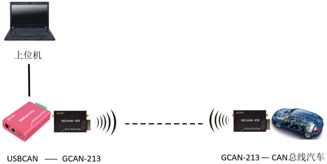
GCAN-213 典型应用 1—移动车辆 CAN-bus 总线调试
