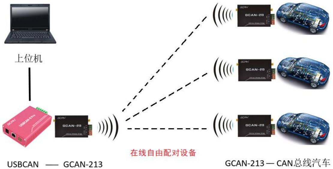
GCAN-213 应用 2—在线自由配对设备
