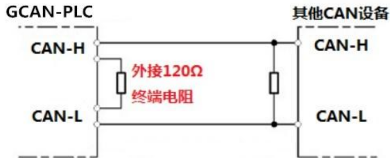
图 3.2 GCAN-PLC-510 与其他 CAN 节点设备连接
