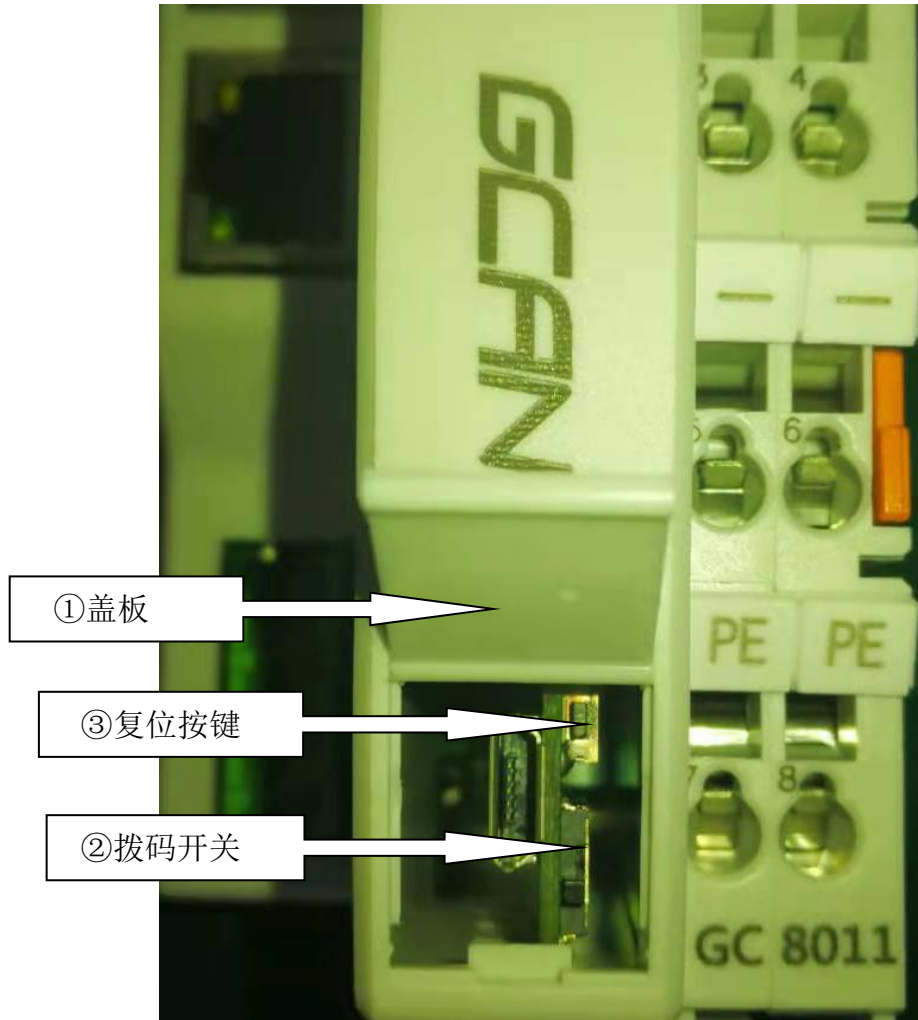
图 4.1 运行开关及复位键实物图
