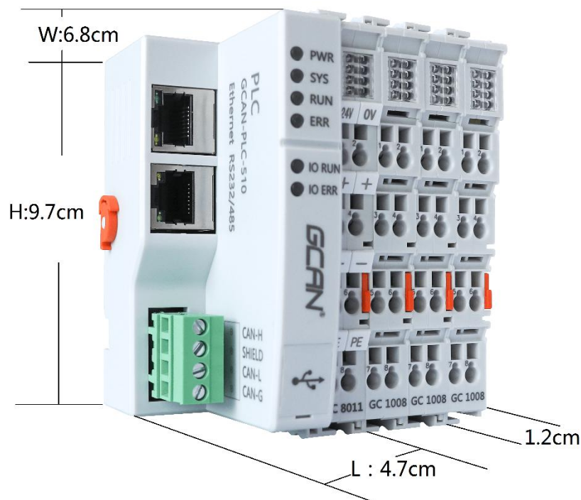
图 2.1 GCAN-PLC-510 外观尺寸图
