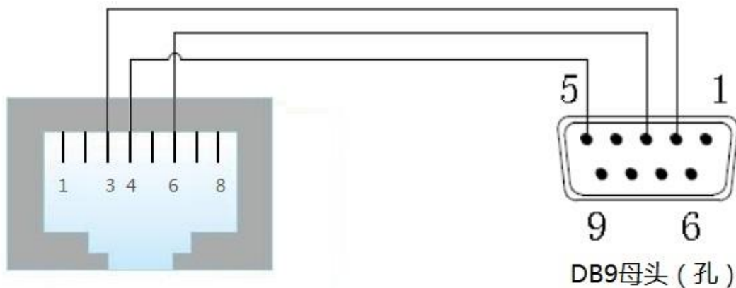
图 2.6 GCAN-PLC-510 的 RS-232 接口样式
