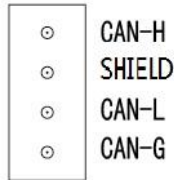
图 2.7 GCAN-PLC-510 的 CAN 总线端子排
