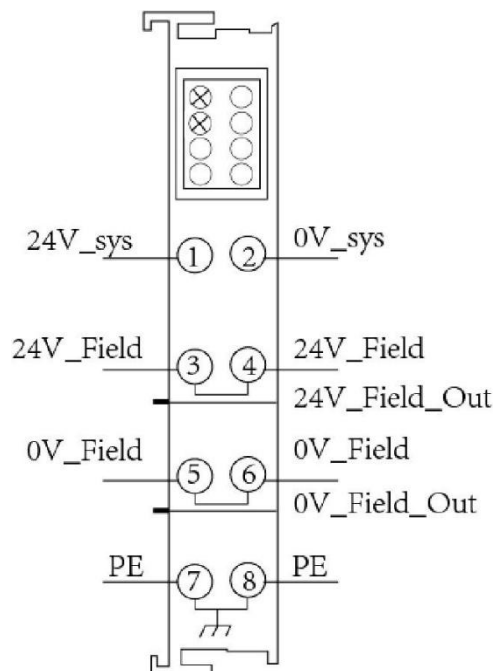
图 2.8 GCAN-PLC-510 电源模块
