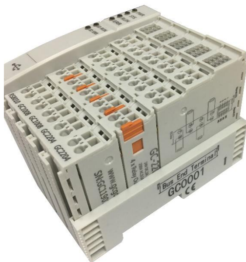
图 2.4 GC-0001 终端电阻模块安装方法
