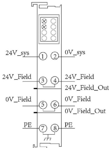
图 2.8 GSCAN-PLC 电源模块
