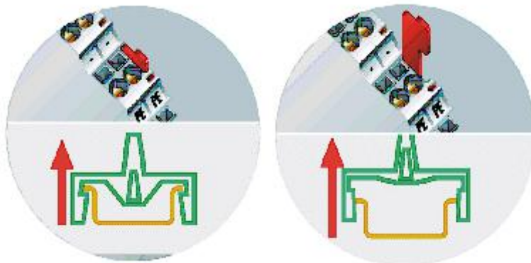
图 2.3 GCAN-PLC 卡扣松脱方式
