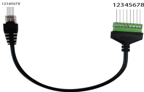
图 2.6 GCAN-PLC-511 的 RJ45 复用接口样式
