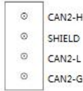
图 2.7 GSCAN-PLC-511 的 CAN2 总线端子排
