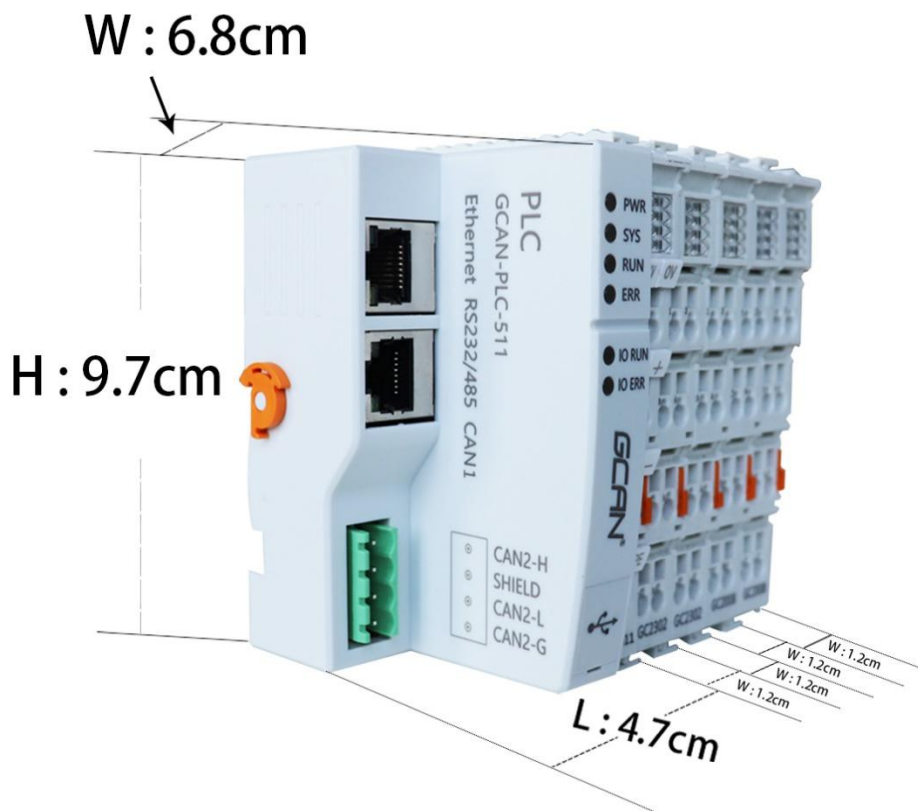
图 2.1 GCAN-PLC 外观尺寸图
