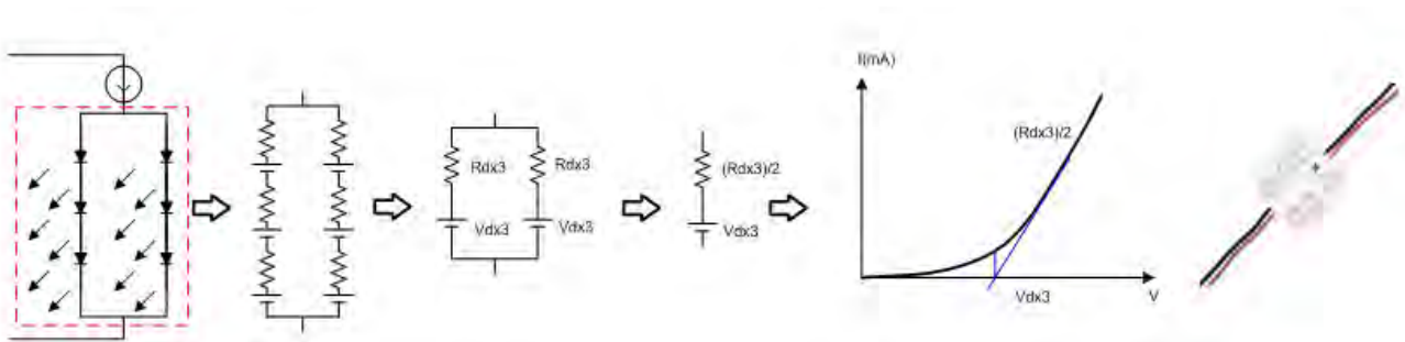
圖 4-11 多個 LED 串並聯等效電路及特性曲線圖
