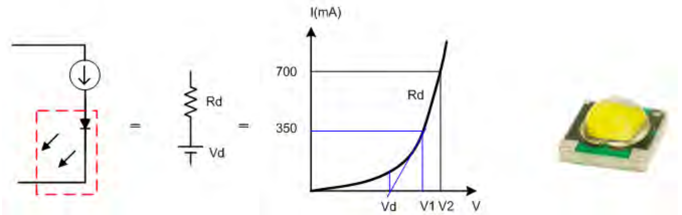
圖 4-8 LED 等效電路及特性曲線圖
