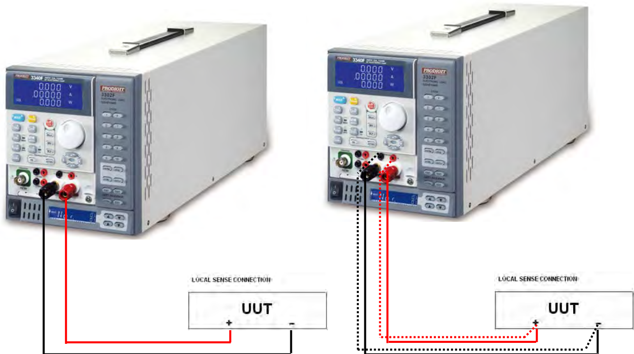
圖 3-2 典型的 3341G 系列電子負載連接方式
