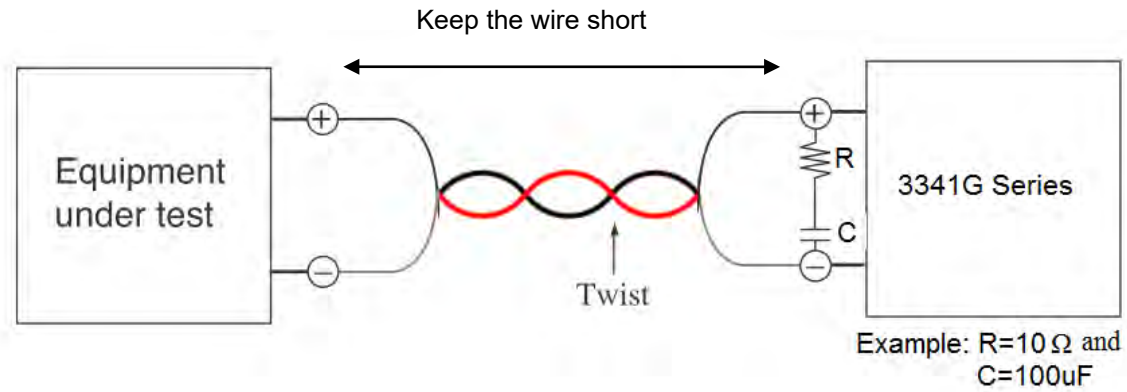
圖 2-5 接線長度
