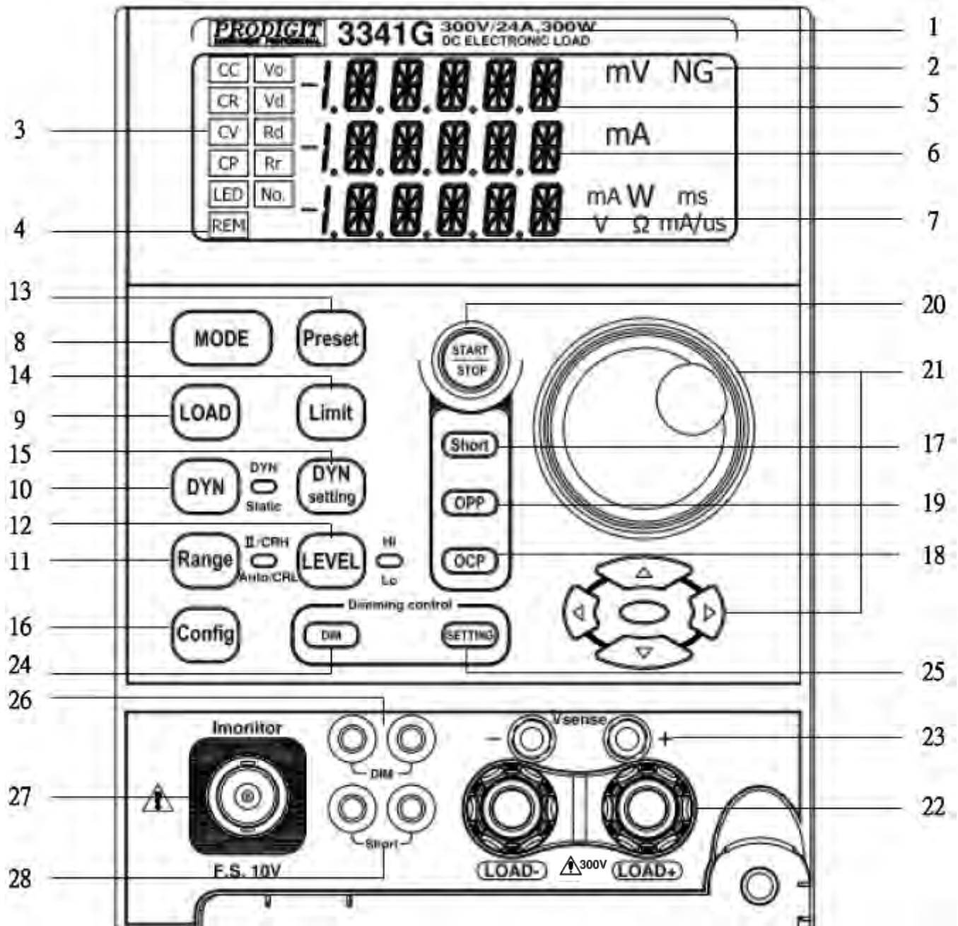
圖 3-1 前面板圖
