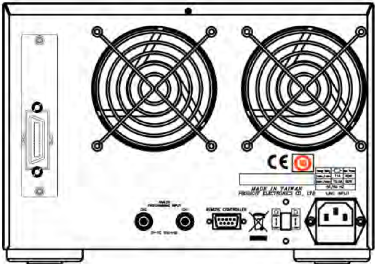
圖 3-3 3305G 後面版圖
