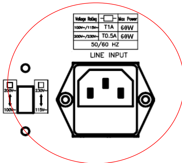
圖 2-1 電源設定圖
