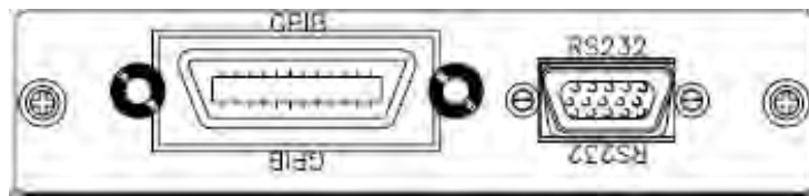
圖 2-3 3305G GPIB & RS232 連接埠圖
