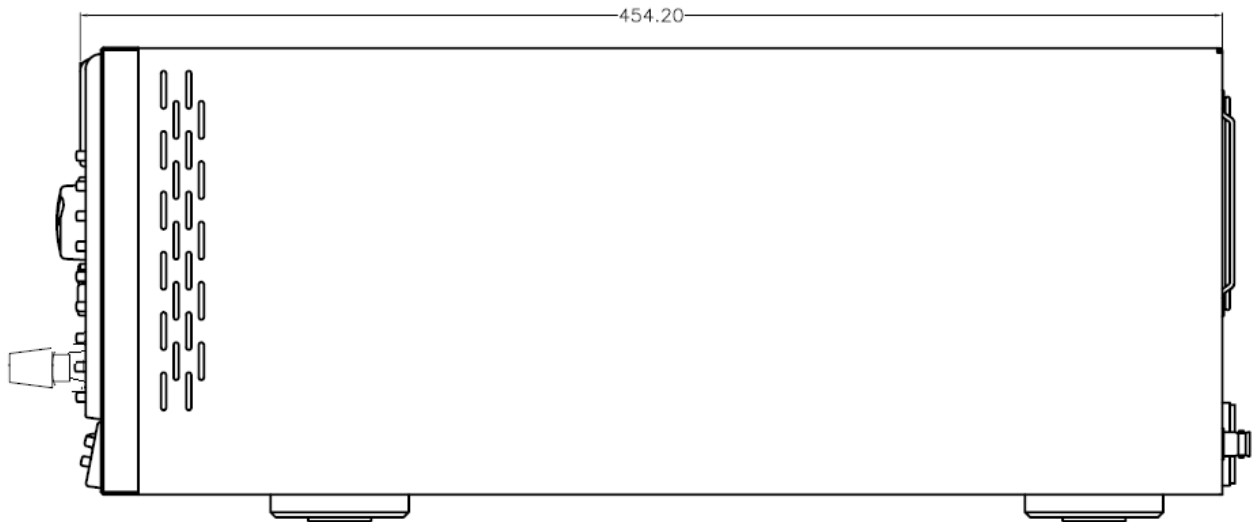
圖 3-2 3302G 側面圖
