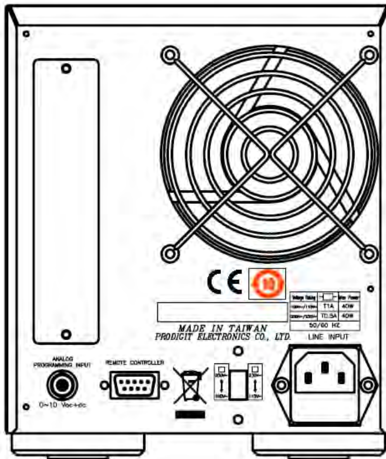
圖 3-3 3302G 後面版圖
