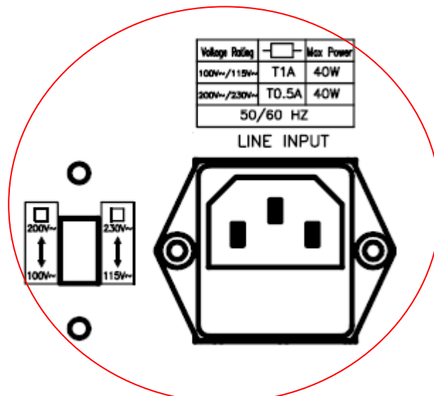
圖 2-1 電源設定圖
