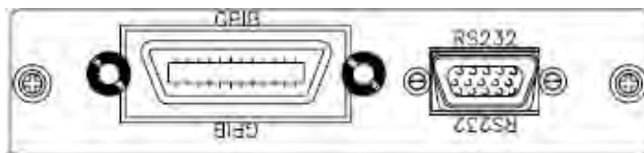
圖 2-3 3302G GPIB & RS232 連接埠圖
