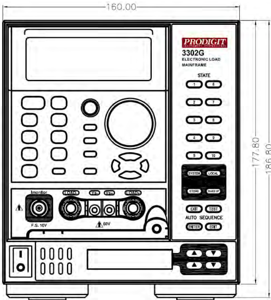
圖 3-1 3302G 前面板圖
