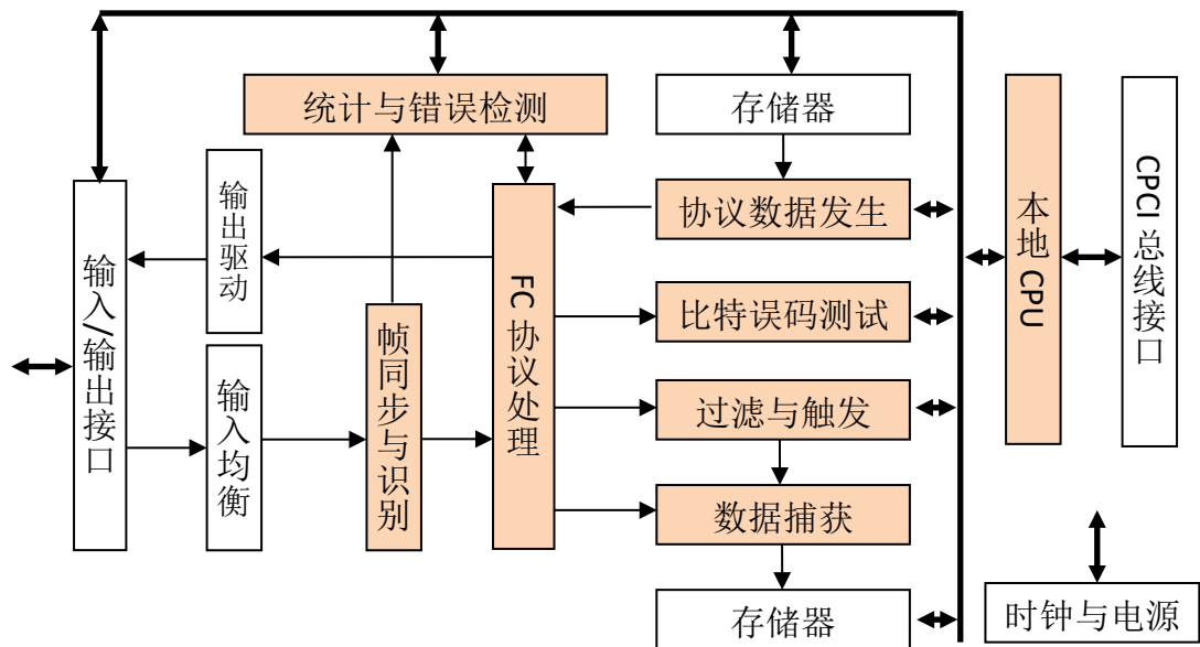
图 3-1 2G FC 总线测试模块原理框图
