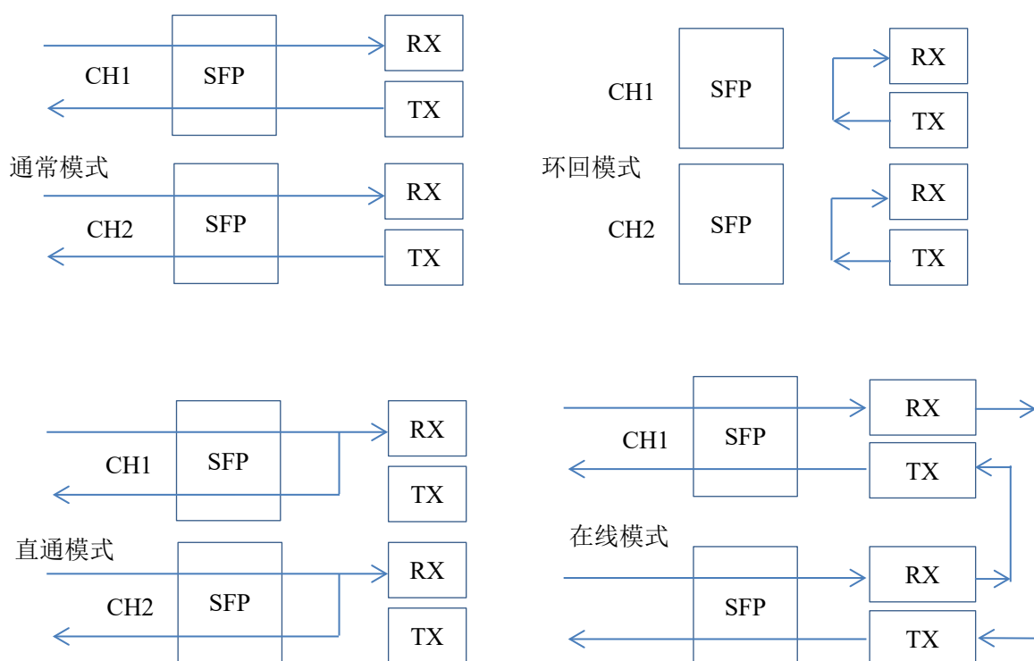
图 2-3 FC 端口模式连接示意图
