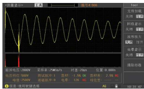
波形正常显示时的电晕显示
