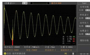
波形放大显示时的电晕显示
