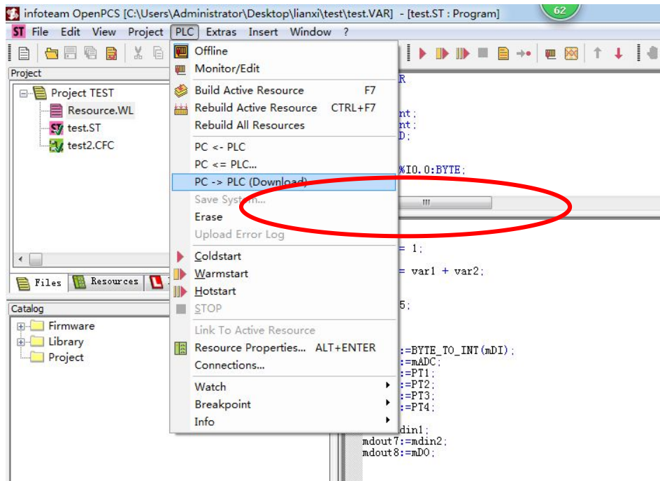
图 4.16 下载程序
