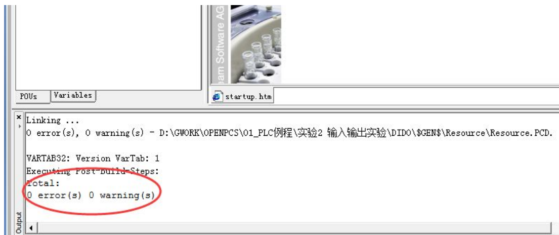
图 4.14 编译完成
