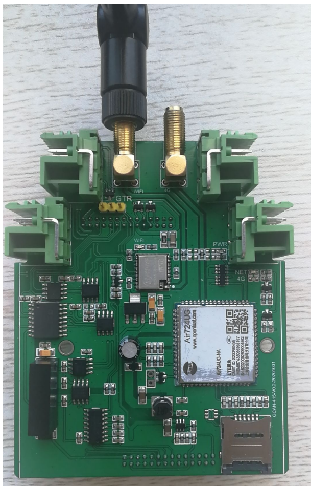
图 3.4 GCAN-GT-415 安装 WIFI 天线
