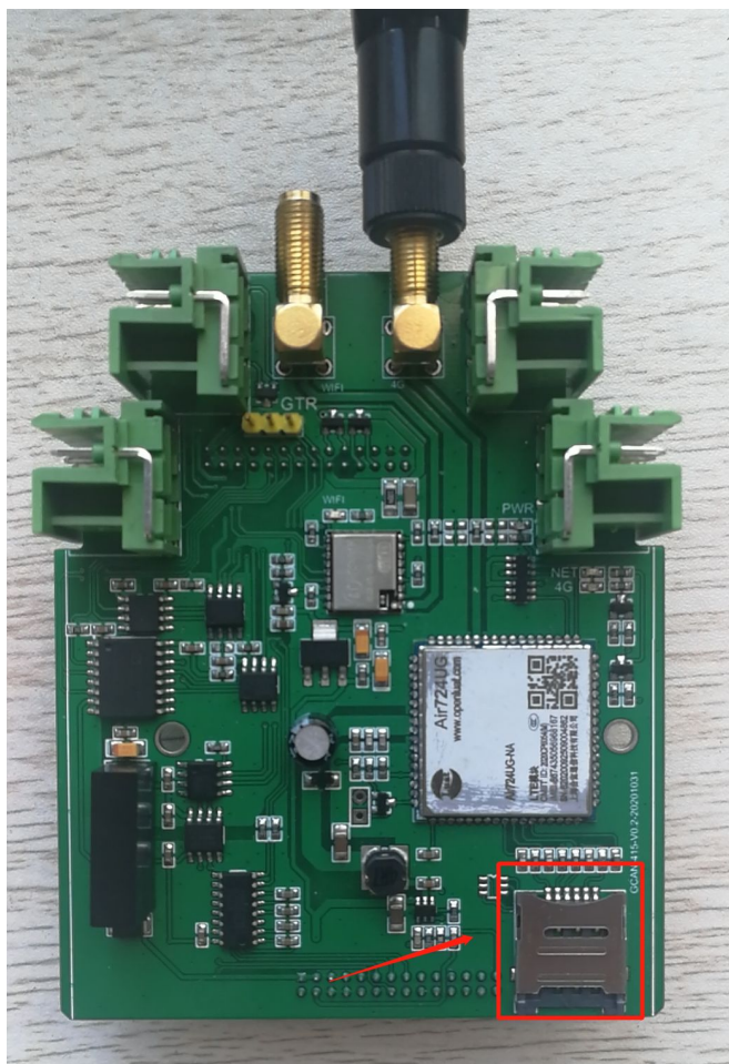
图 3.3 GCAN-GT-415 安装 4G 天线及 4G 卡
