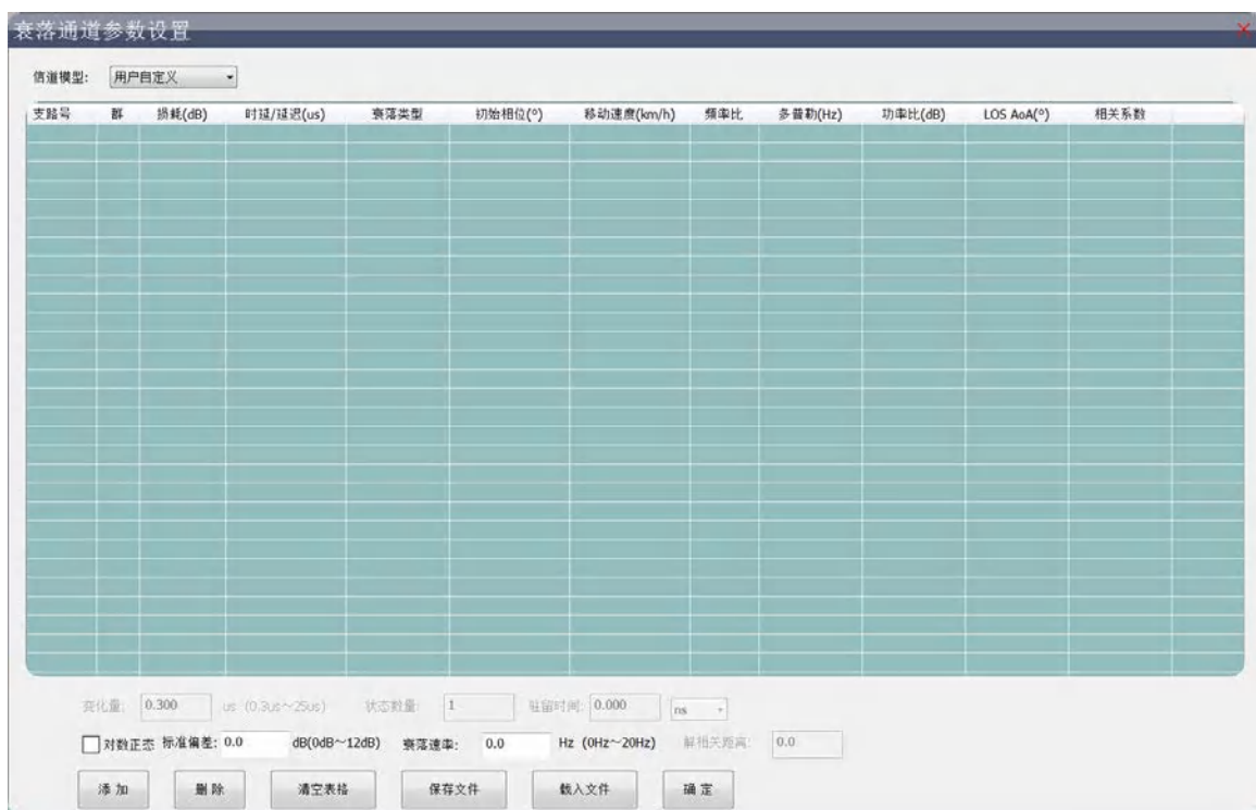
图 3.17 衰落通道参数设置
