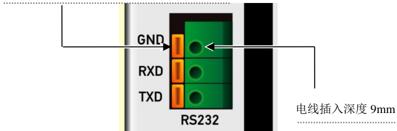
图 5-3 IPMP 系列远端补偿接口
