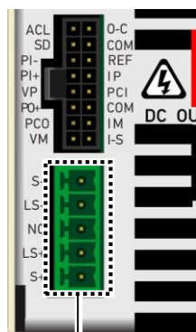
电压补偿端子接口 J4
