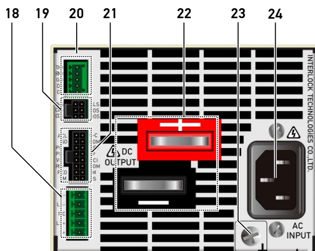
图 2-2 IPX（低压大电流）系列后面板
