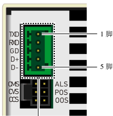
RS232 和 RS485 接口
