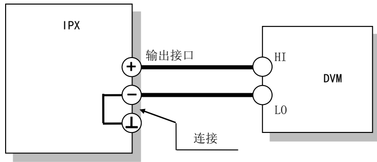
图 7-4 电压校准连接
