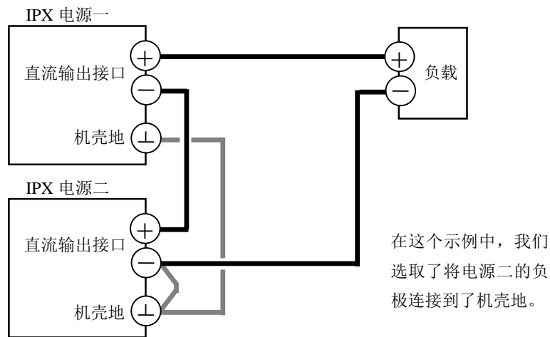
图 3-5 串联模式的负载连接
