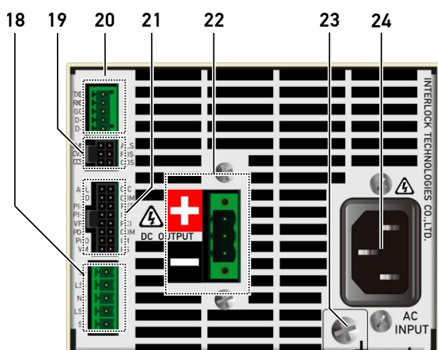
图 2-3 IPX（中高压小电流）系列后面板
