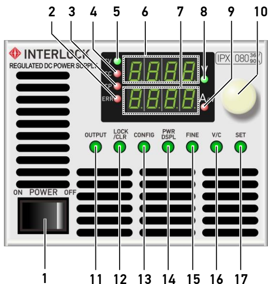
图 2-1 IPX 系列前面
