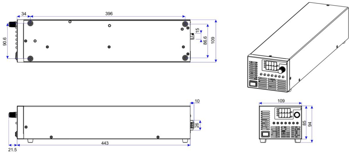
IPX 系列 中高压小电流外观和尺寸 b 示意图
