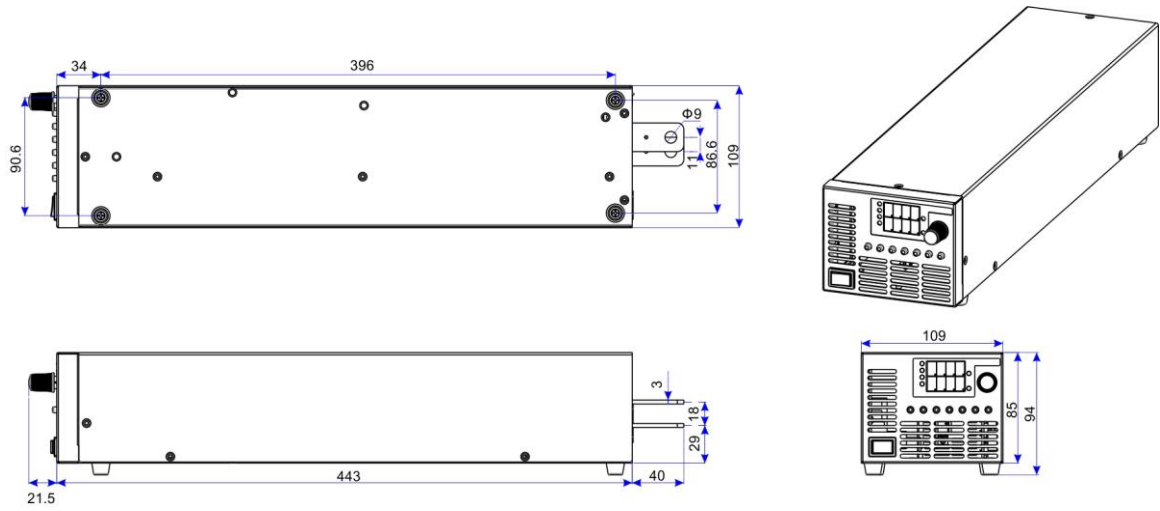
IPX 系列 低压大电流外观和尺寸 a 示意图
