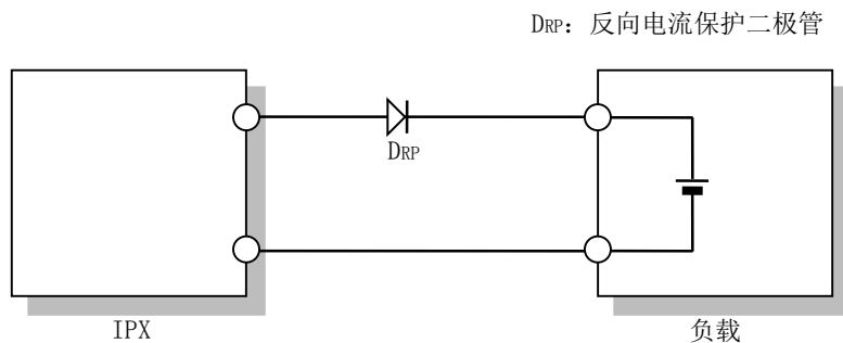
图 3-9 储能负载的连接方法
