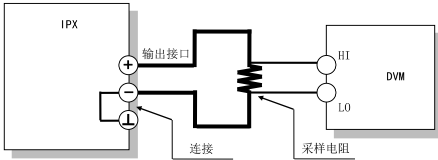
图 7-5 电流校准连接
