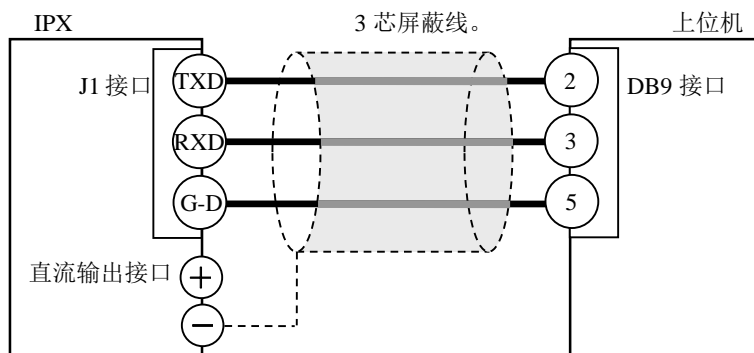
图 7-2 RS232 接口连接示意图
