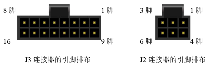
图 5-4 用户正视后面板时的引脚分布图
