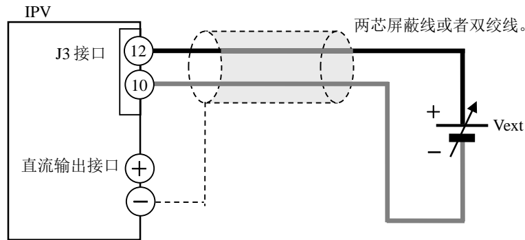
图 5-7 外部控制电压连接示意图
