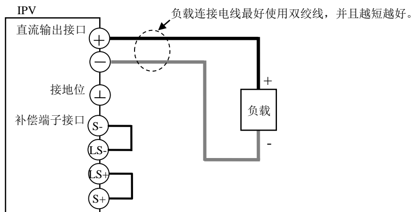
图 3-5 本地电压补偿模式
