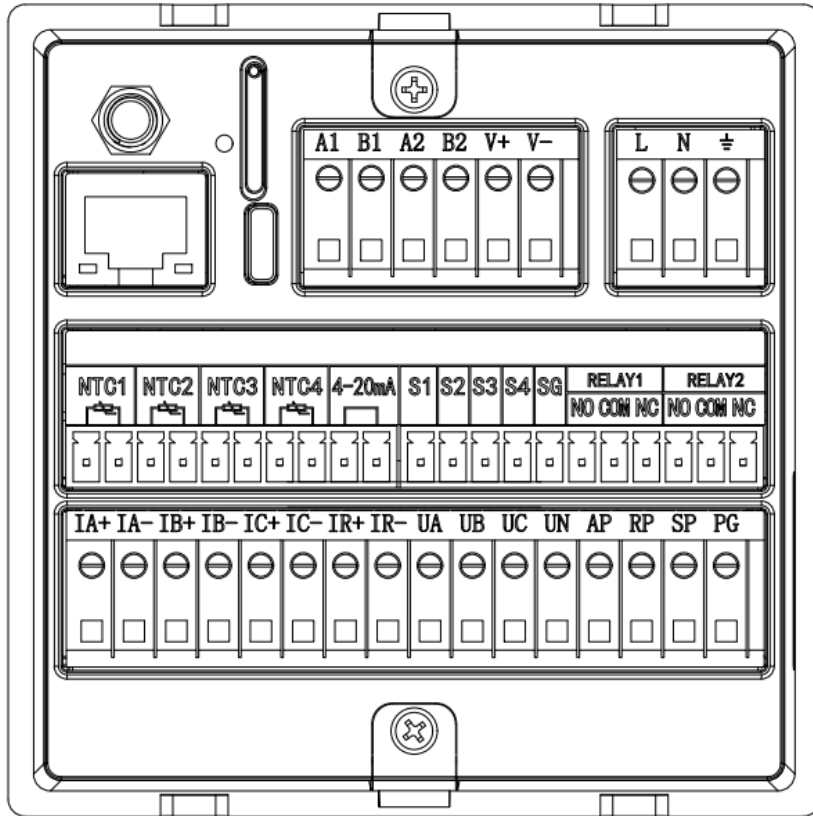
方式1 (3个CT): 三相四线的接线方式
