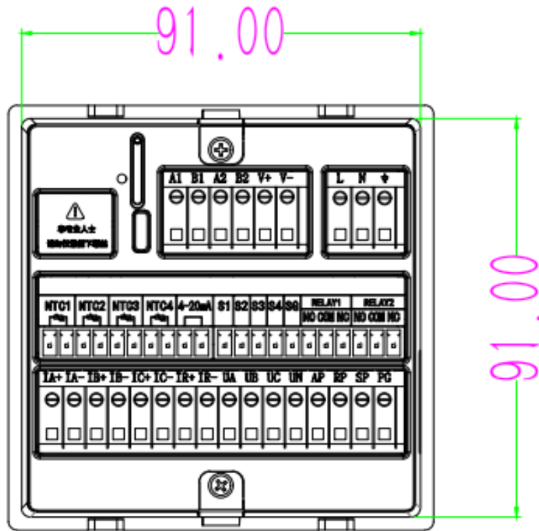
背面尺寸图
