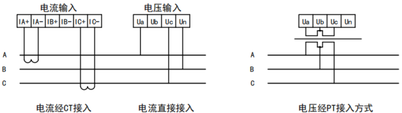
方式2 (2个CT): 三相三线的接线方式
