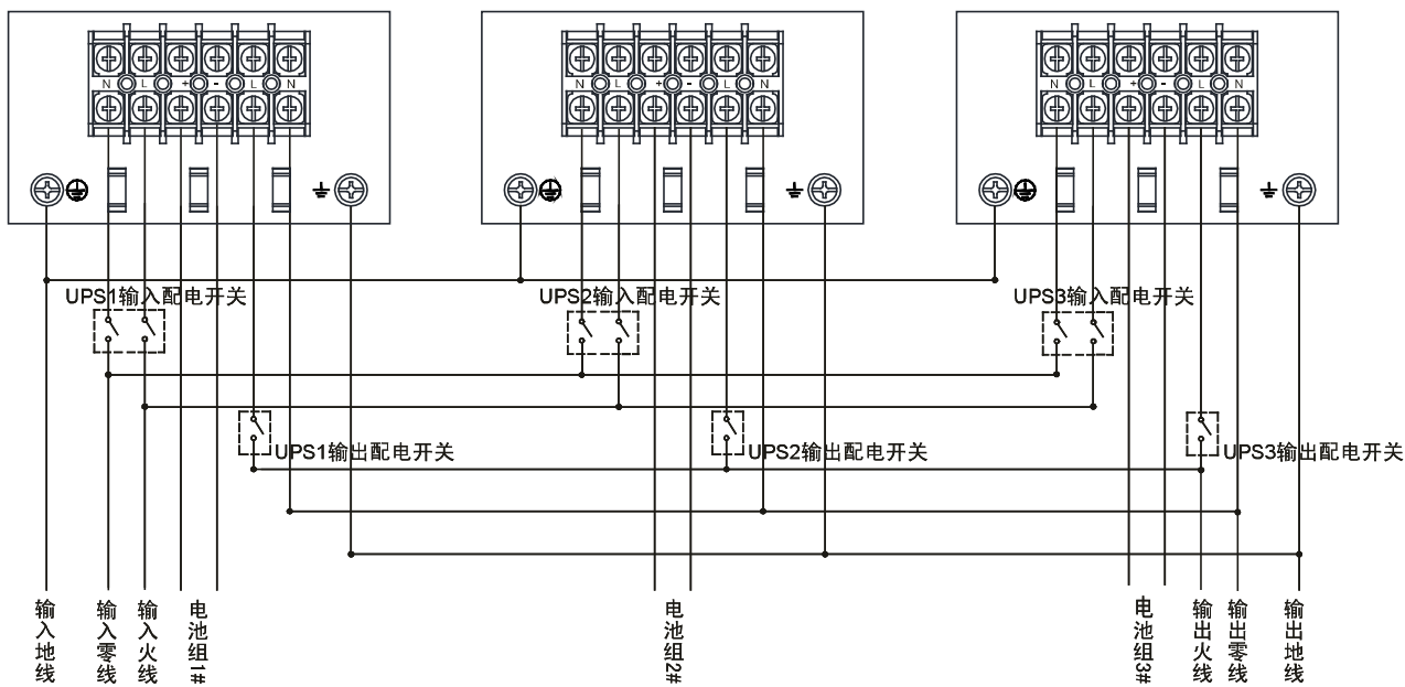
C6KS/C10KS并机接线图
