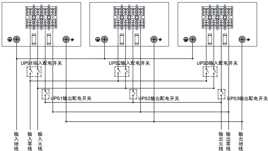
C6K/C10K并机接线图
