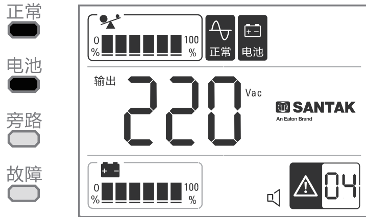
(电池工作模式)
