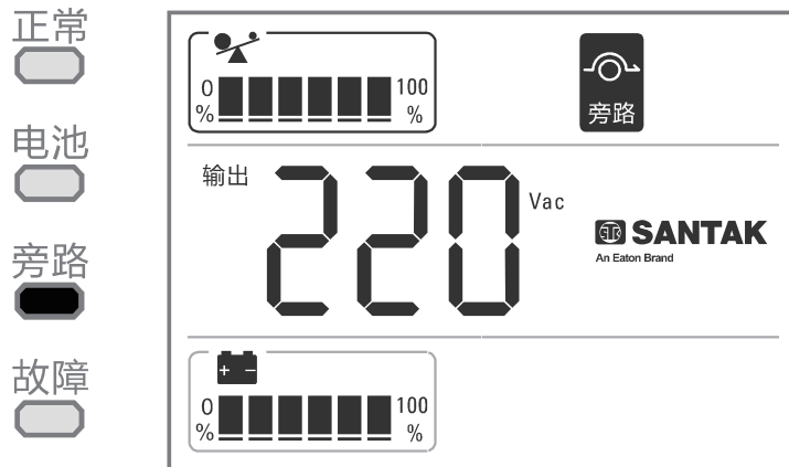
(旁路工作模式)
