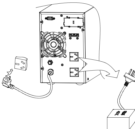
C1K(S)~C3K(S)输出接线方式
