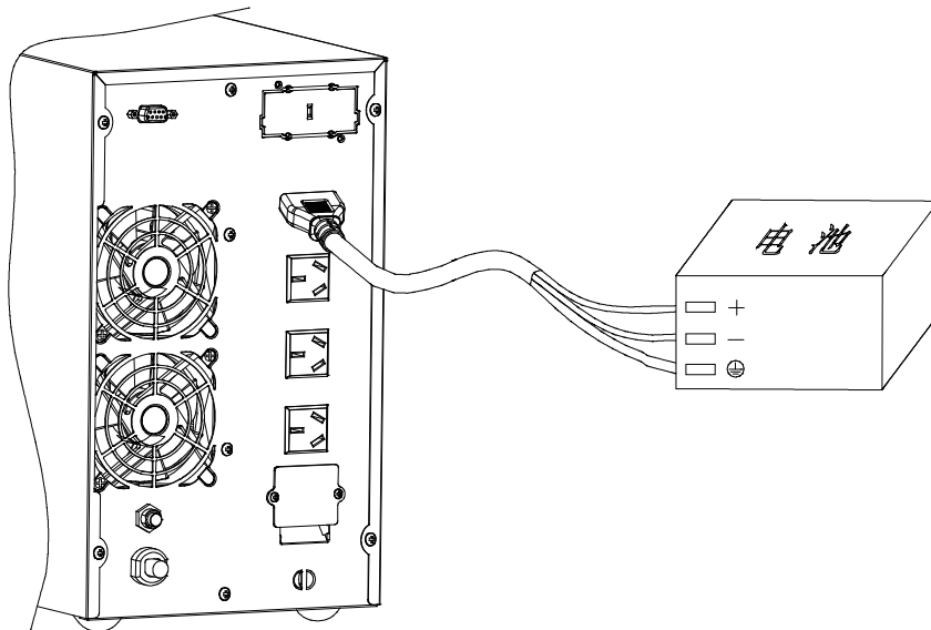
长效型UPS电池连接示意图
