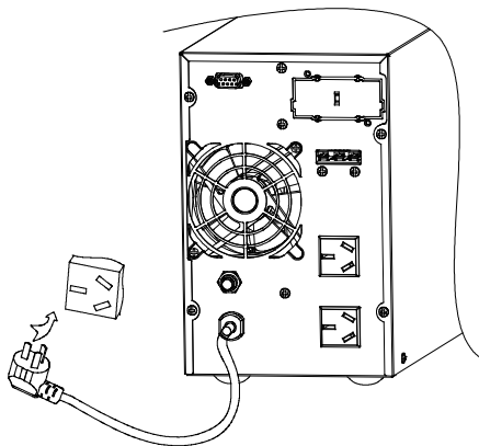
C1K(S)~C3K(S)输入接线方式
