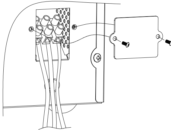
C3K(S)端子排连接方式
